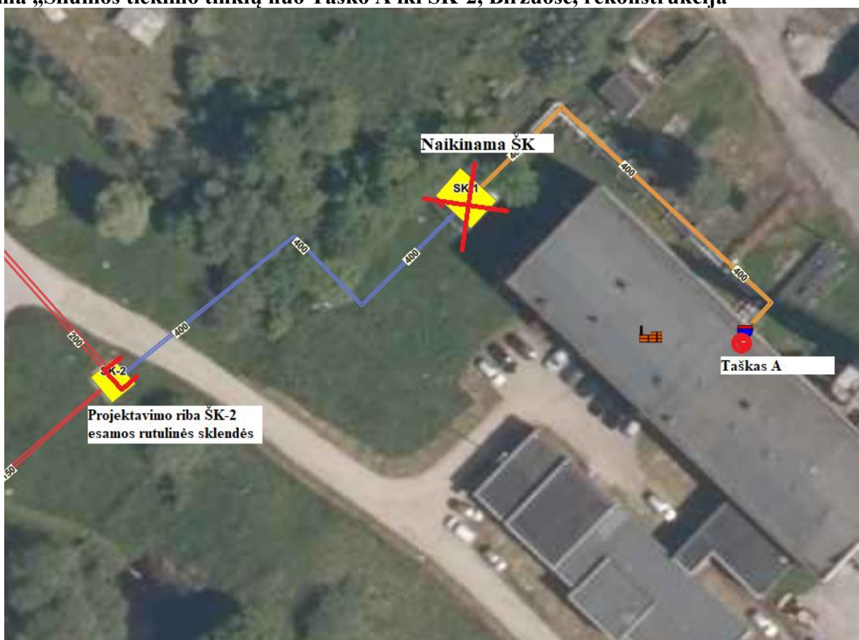
1 schema „Šilumos tiekimo tinklų nuo Taško A iki ŠK-2, Biržuose, rekonstrukcija“
