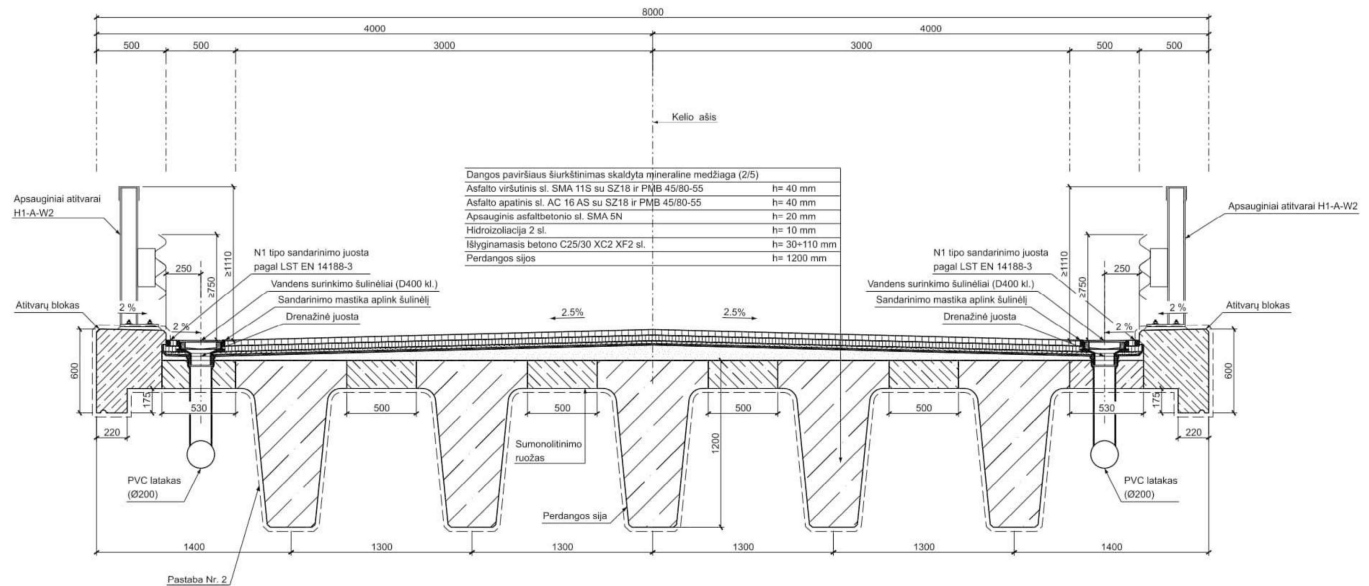
Pav. 1 Tilto skersins pjūvis
