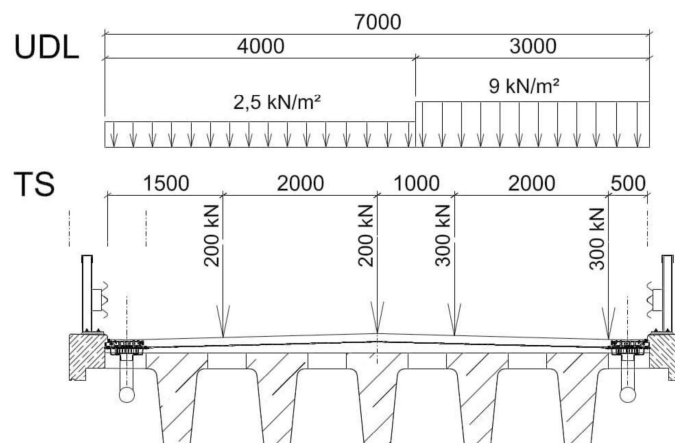
Pav. 4 Automobilių eismo kintamų apkrovų išdėstymo schema
