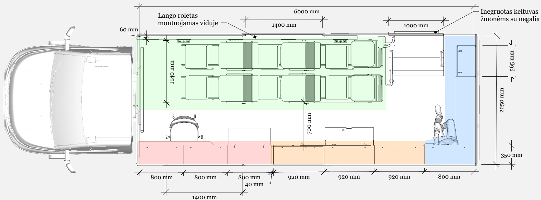
BALDŲ IR INVENTORIAUS IŠDĖSTYMO PLANAS:
