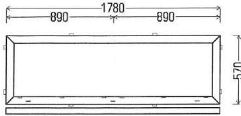
Vaizdas iš vidaus V2 (16vnt)
