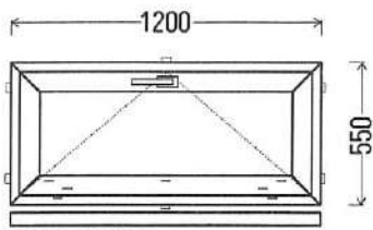
Vaizdas iš vidaus L1 (1vnt)
