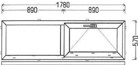
Vaizdas iš vidaus L3 (2vnt)
