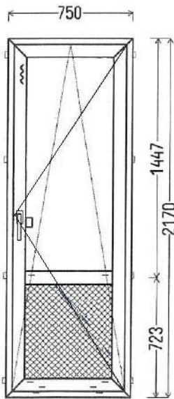
Vaizdas iš vidaus BD5 (7vnt)
