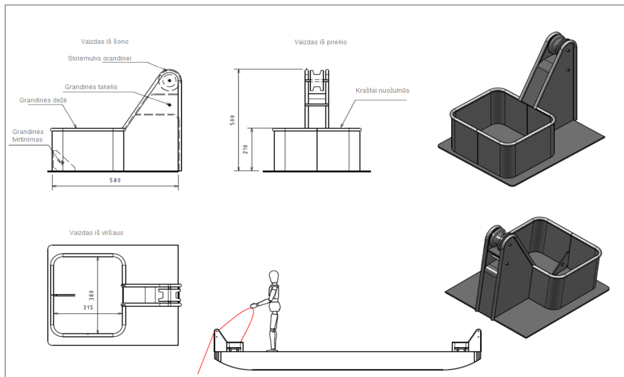
2 pav. Galimas Kelto per Aiseto ežerą varymo mechanizmas
