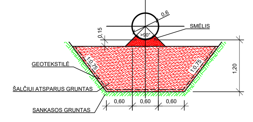
Pjūvis 2-2
