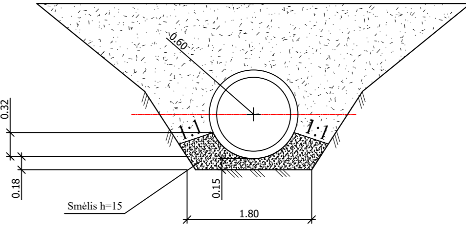
Pjūvis 2-2
