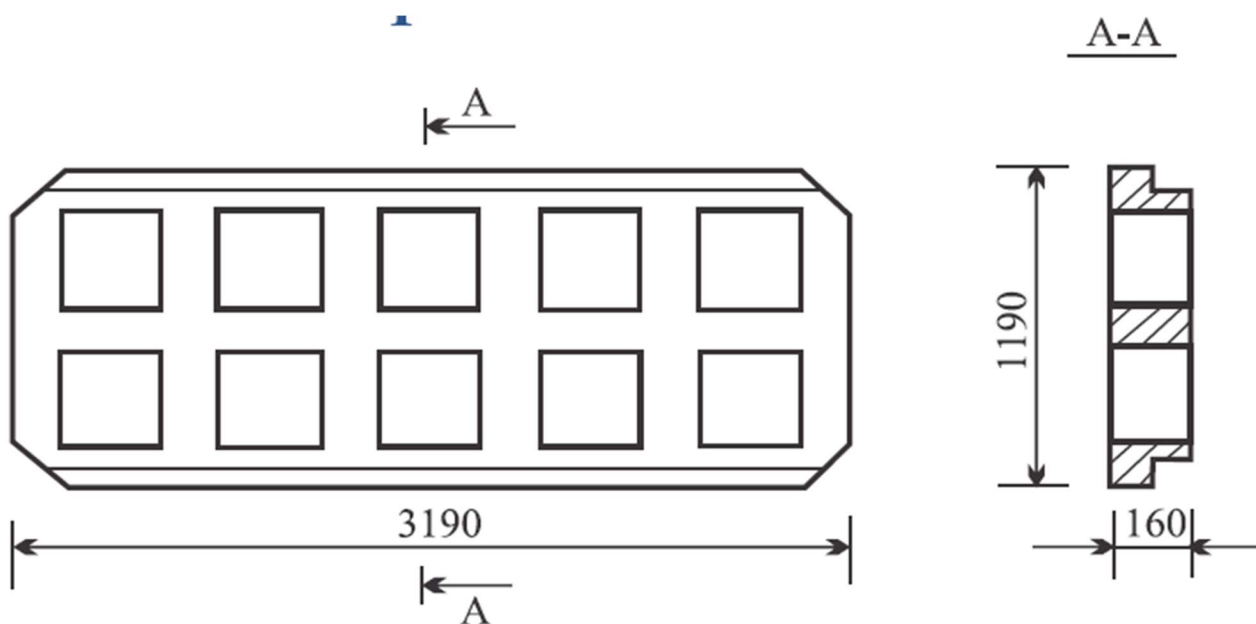
Pav. 1. Šlauto tvirtinimo plokštė PR-1.
