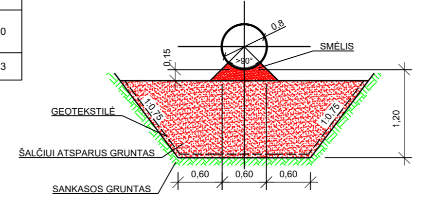
PJŪVIS 1-1
