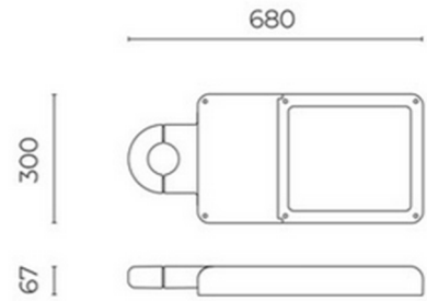
3 pav. Šviestuvo matmenys
