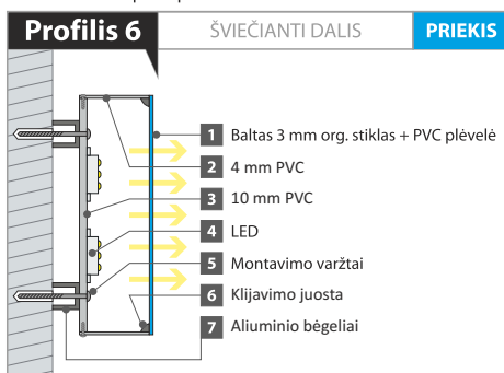
Tūrinės iškabos principinė schema
