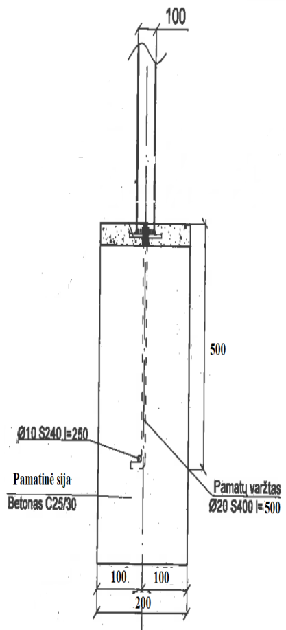
Plieninė plokštė, virinama prie metalinės kolonos, skirta tvirtinimui prie pamatinės sijos
