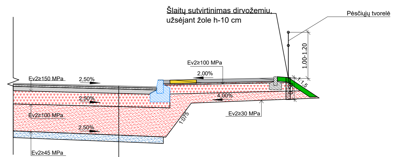
Autobusų stotelės skersinis profilis
