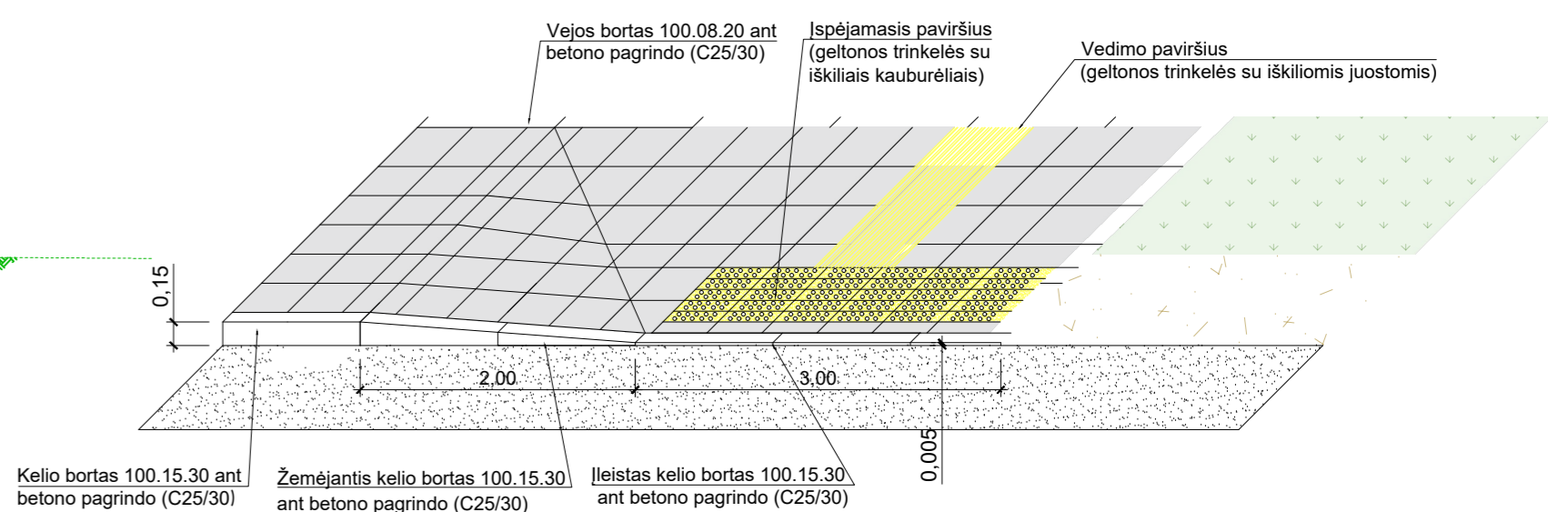
Autobusų stotelės skersinis profilis
