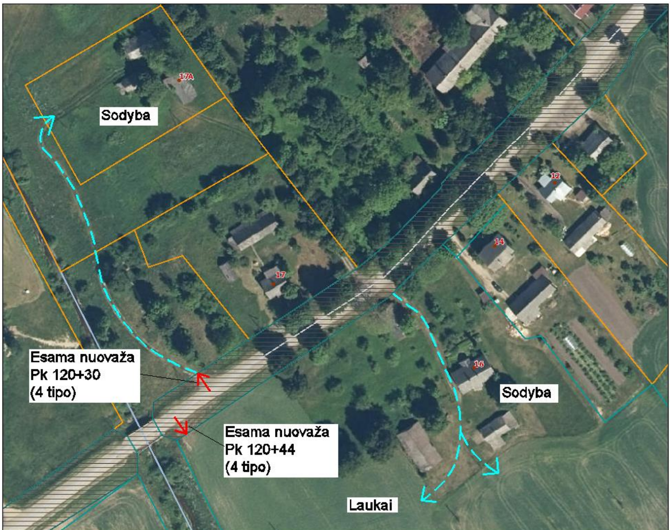
3 pav. Nuovažų esamos situacijos schema.
