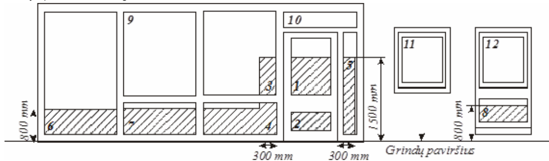
1 pav. Sienose esančių langų ir išorinių durų įstiklinimo padėty. Užstrichuotos zonos 1, 2, 3, 4, 5, 6, 7, 8 parodo kritines įstiklinimo padėtis.
