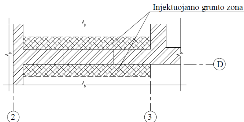
STIPRINAMŲ PAMATŲ SCHEMA M 1:150
