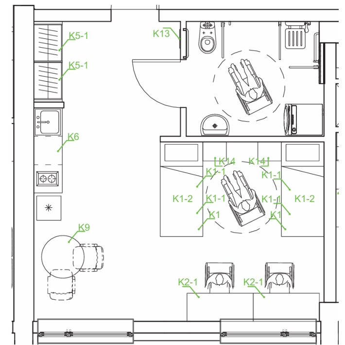
NĖ Neįgaliųjų poreikiams pritaikytas blokas
