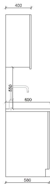
VAIZDAS IŠ ŠONO
