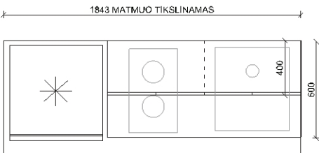
VAIZDAS IŠ VIRŠAUS
