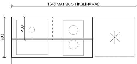
VAIZDAS IŠ VIRŠAUS
