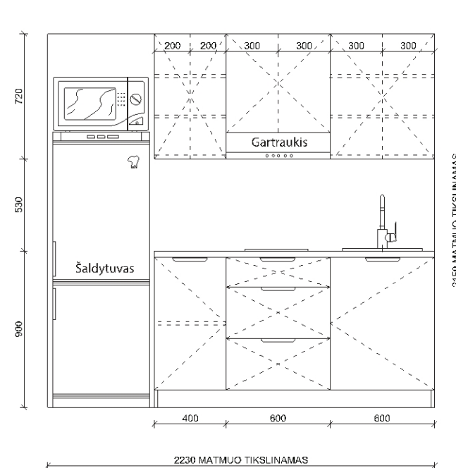
VAIZDAS IŠ PRIEKIO
