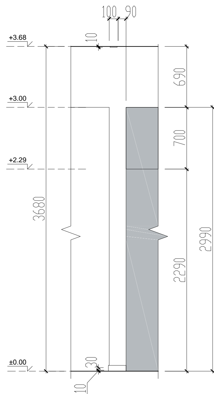
VITRINOS VD 1 MONTAVIMO VIETOS ESAMOS SITUACIJOS APMATAVIMŲ PJŪVIS M1:25
