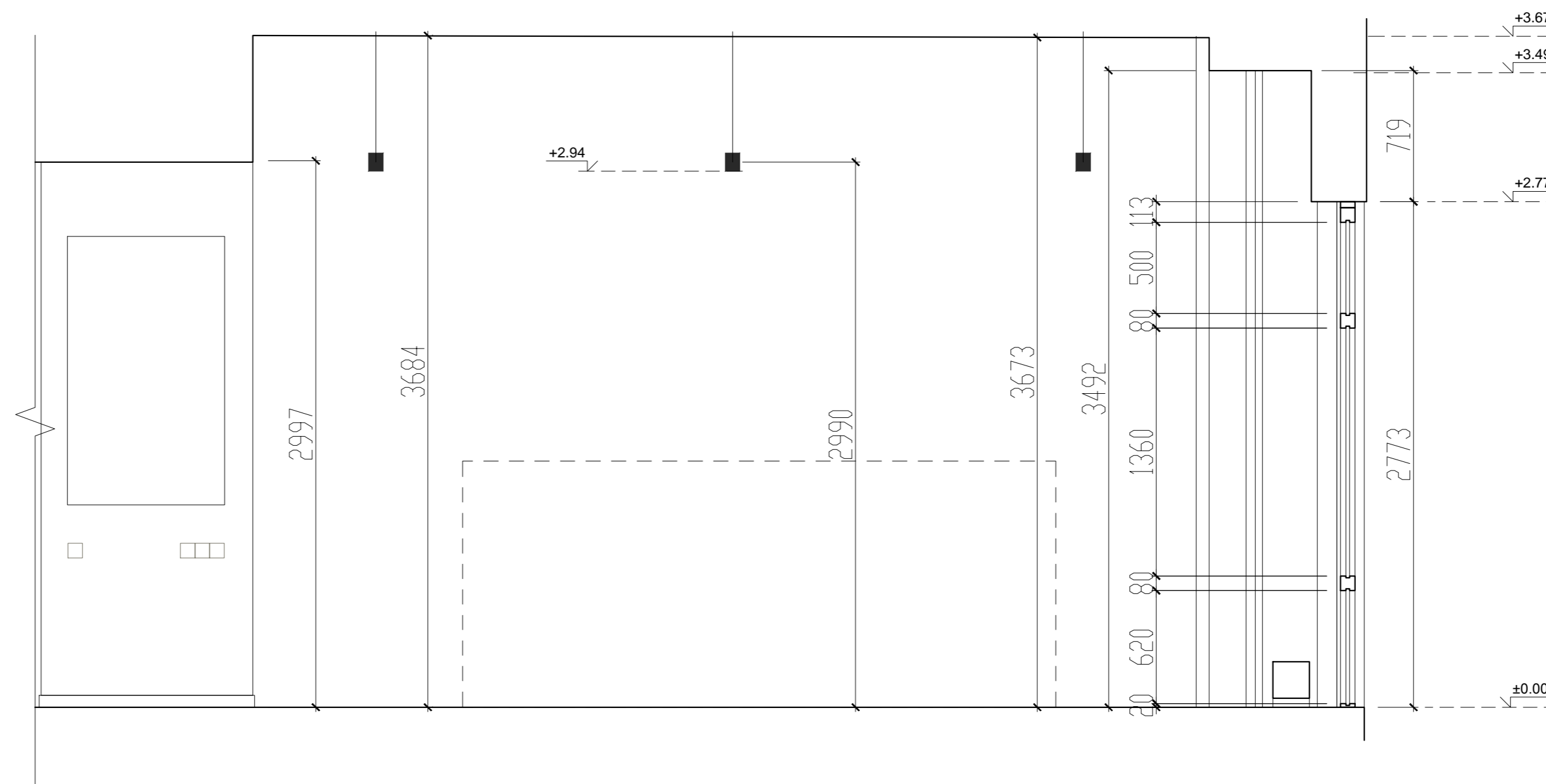
VITRINOS VD 1 MONTAVIMO VIETOS ESAMOS SITUACIJOS APMATAVIMŲ PJŪVIS M1:25
