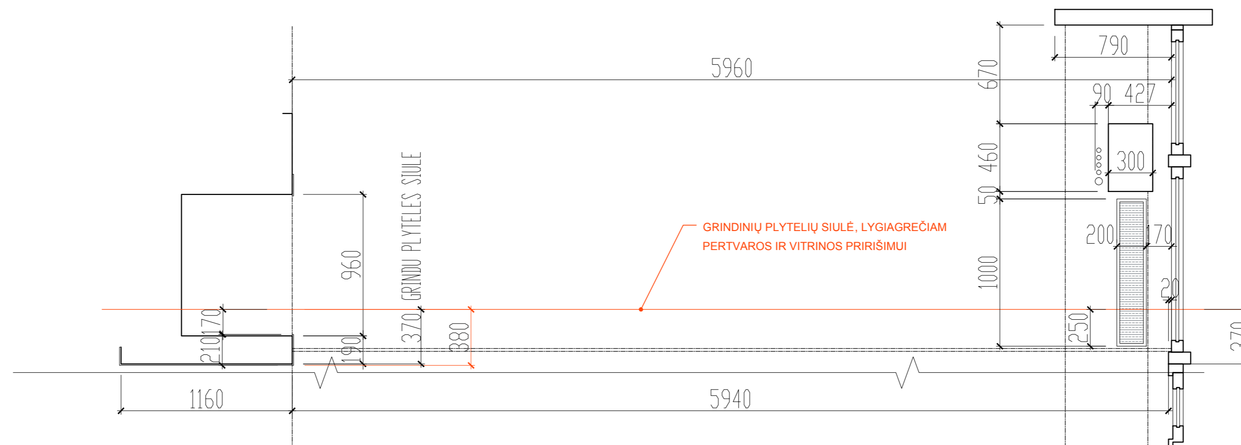
VITRINOS VD 1 MONTAVIMO VIETOS ESAMOS SITUACIJOS APMATAVIMŲ PLANAS M1:25
