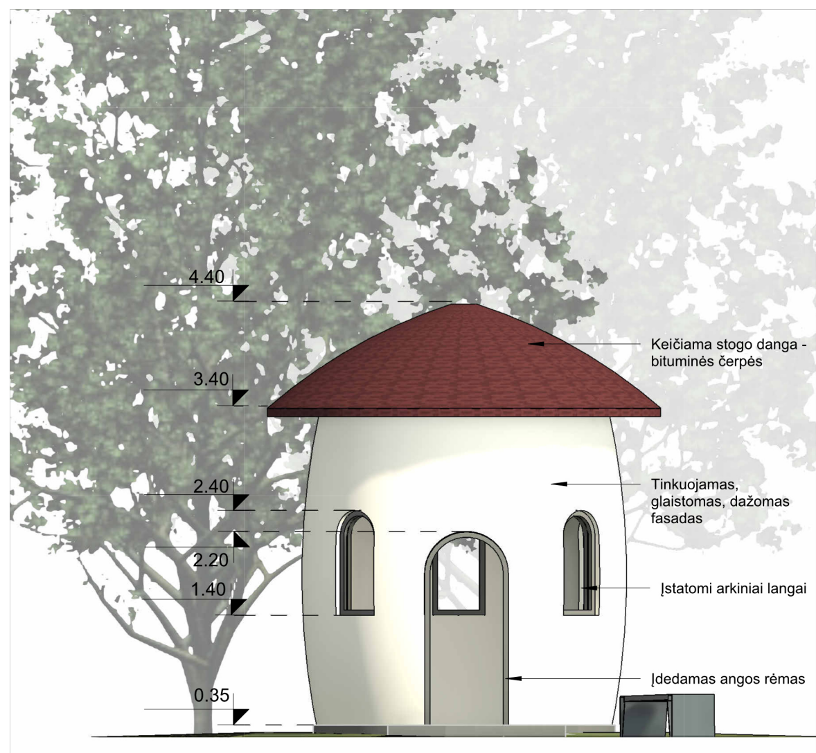
Pavėsinės "grybuko" išklotinė
