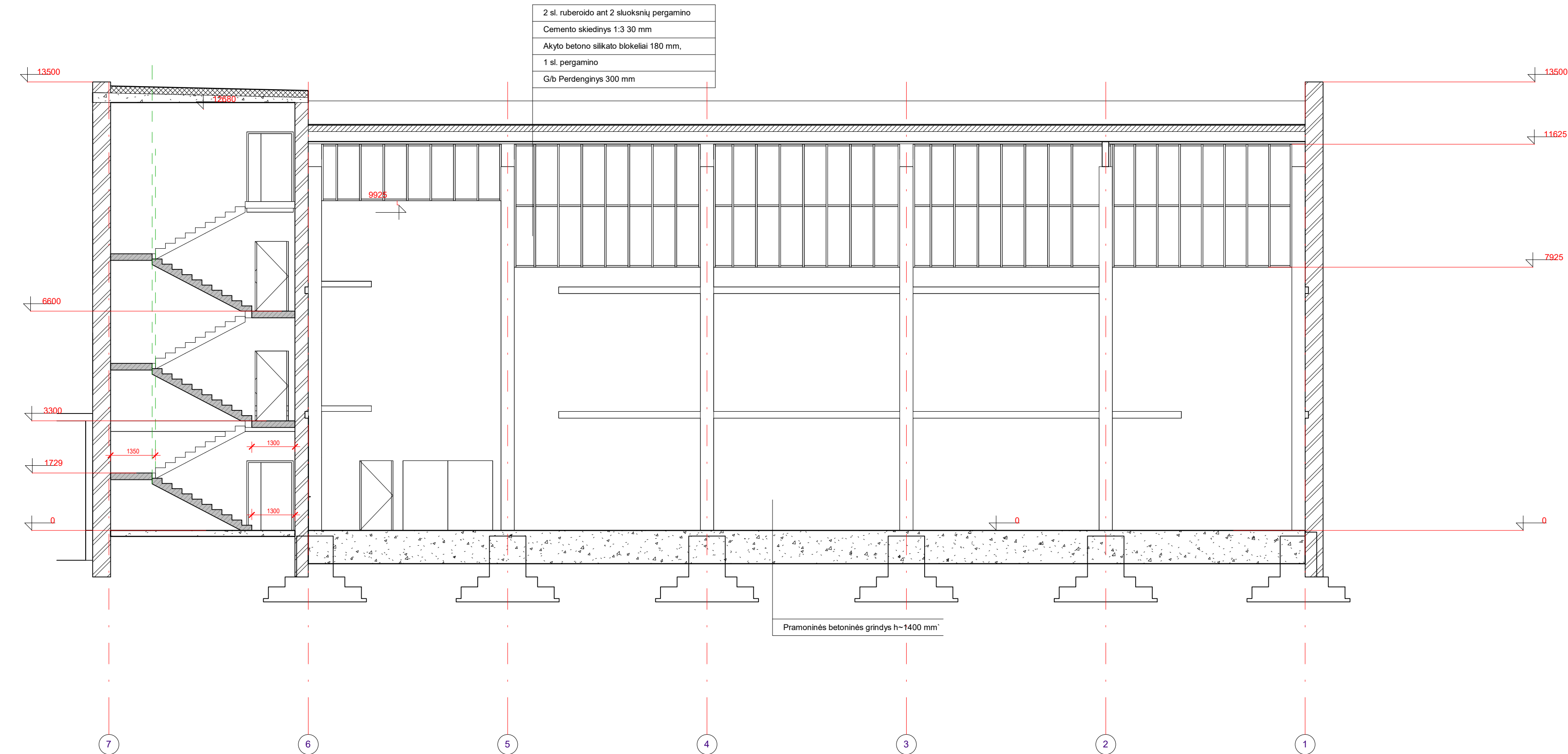
PJŪVIS D-D
