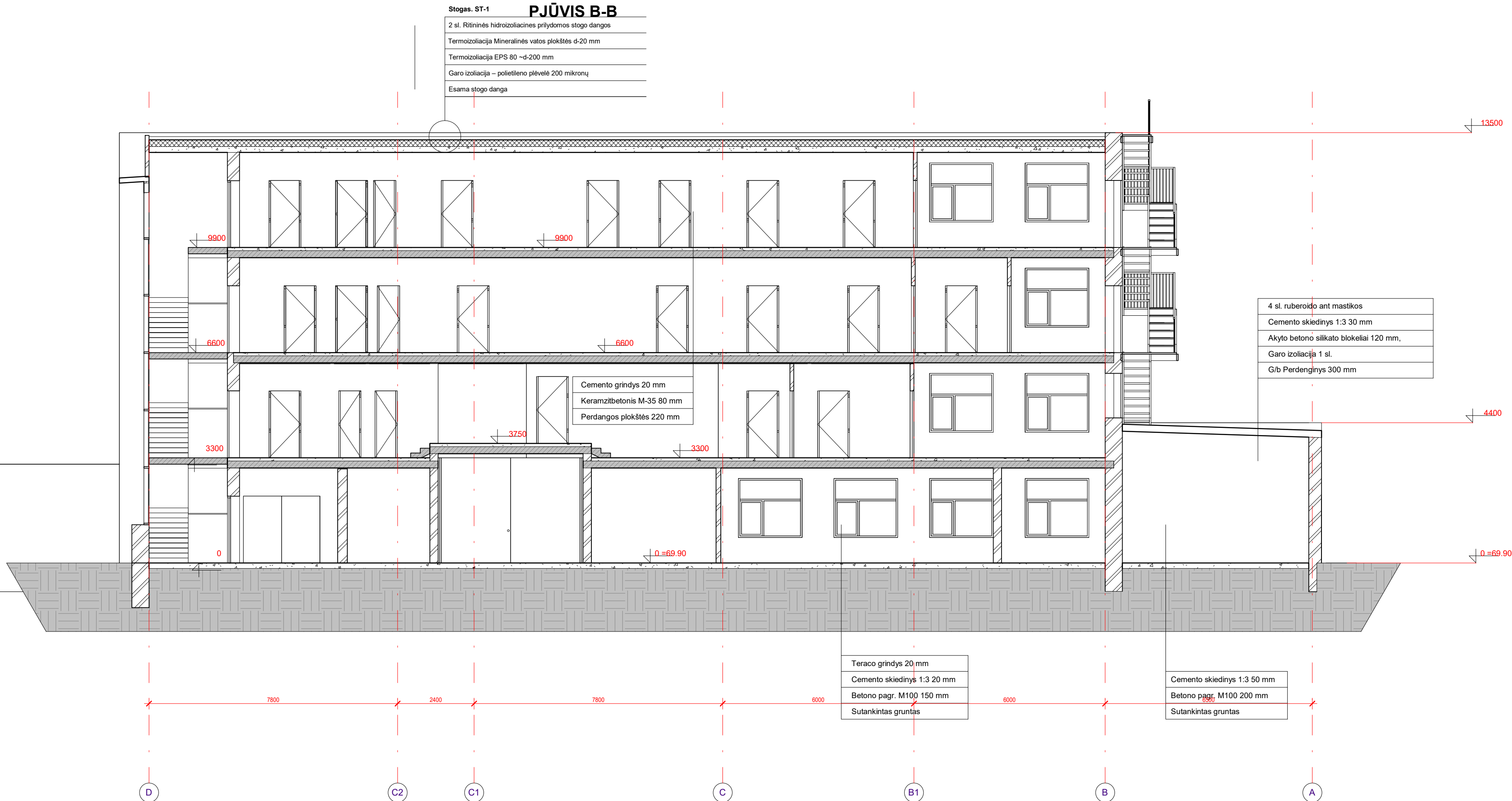
PJŪVIS B-B
