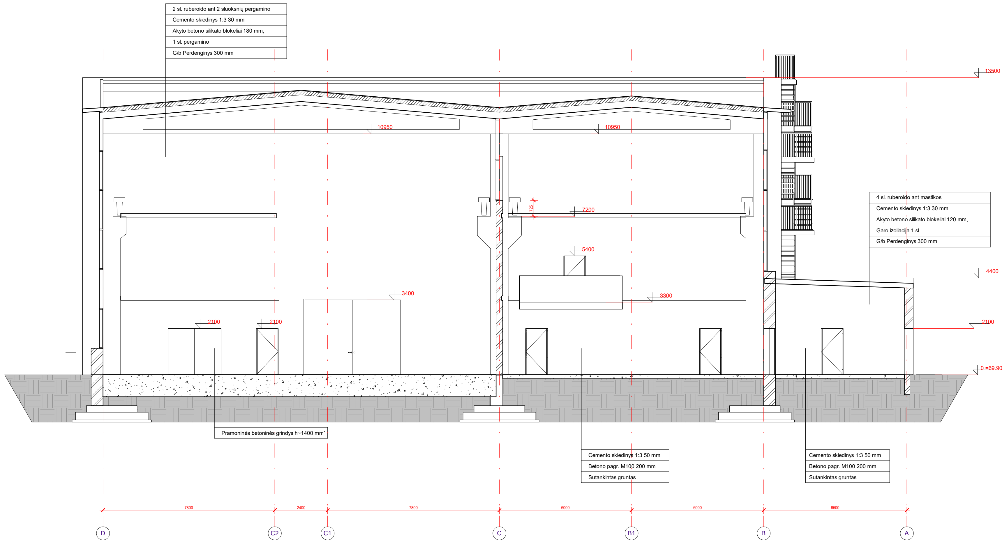
PJŪVIS B-B
