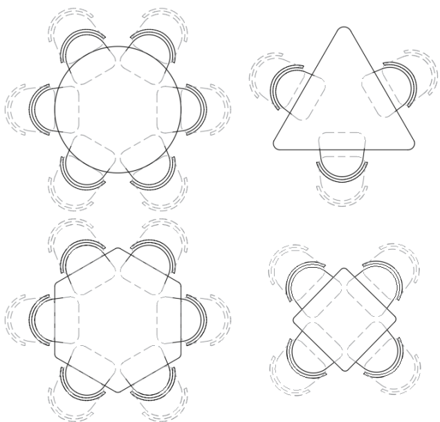
REGULIUOJAMO AUKŠČIO STALIUKŲ FORMOS
