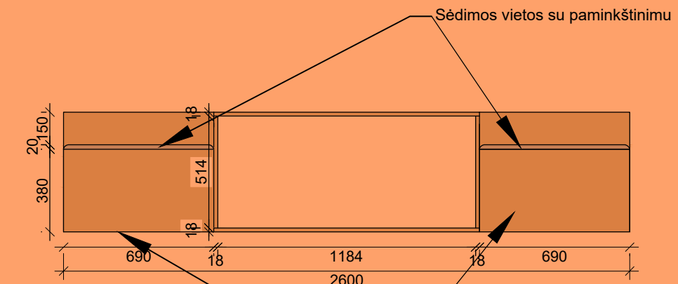
Išklotinė B-B
