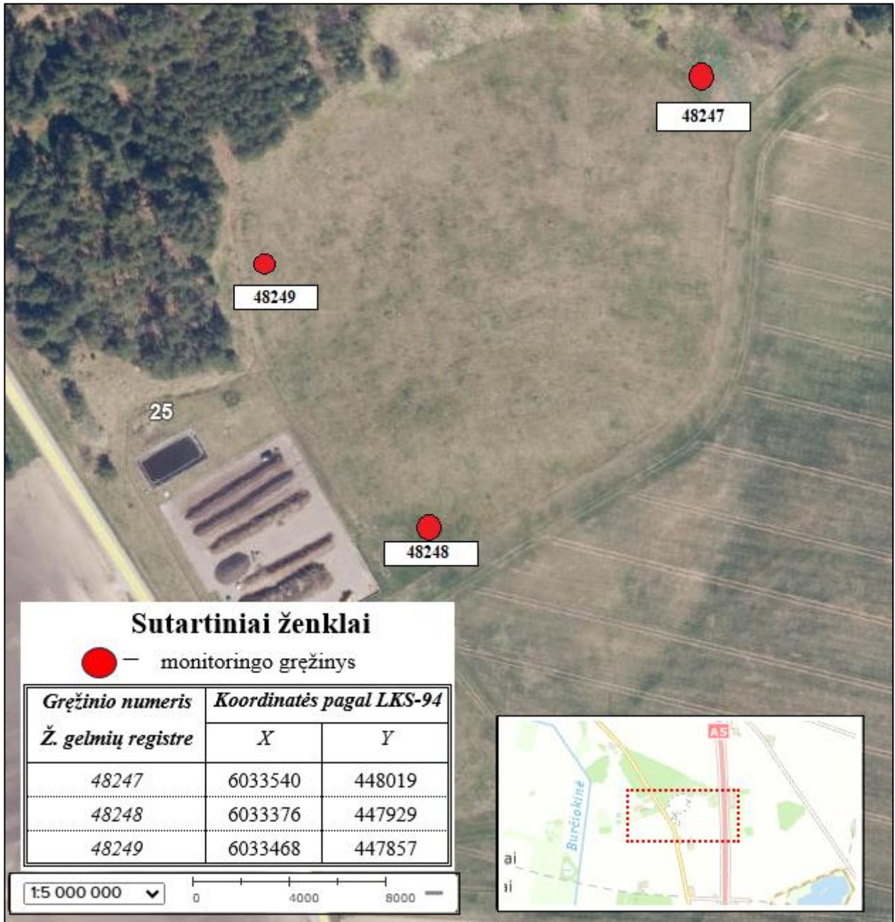
2 pav. Poveikio požeminiam vandeniui monitoringo tinklo schema
