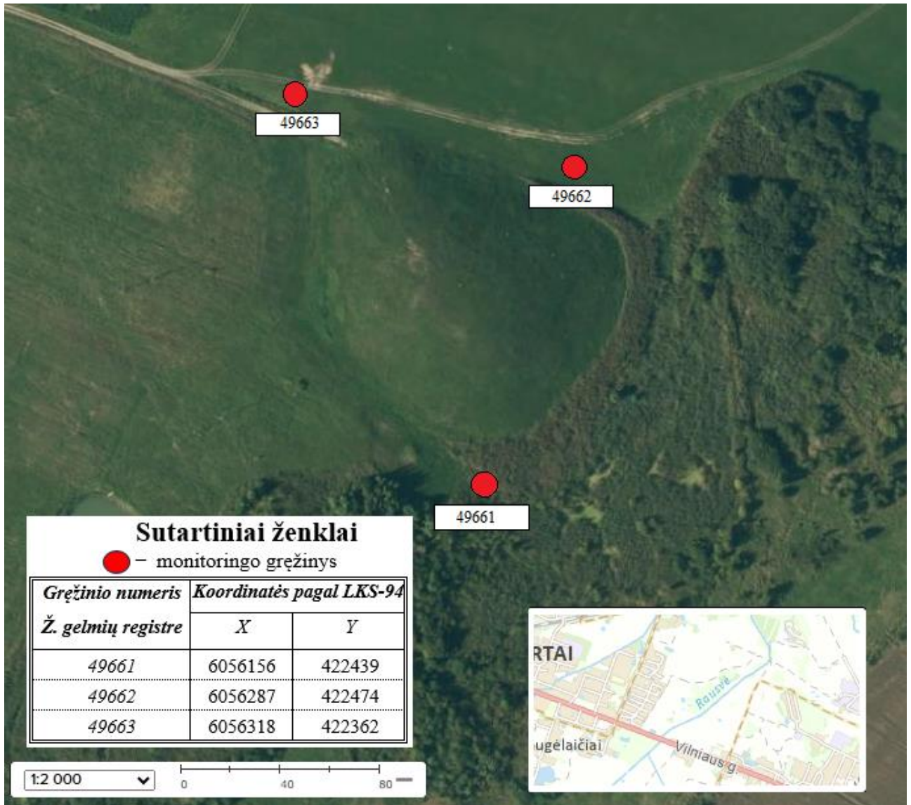
2 pav. Poveikio požeminiam vandeniui monitoringo tinklo schema
