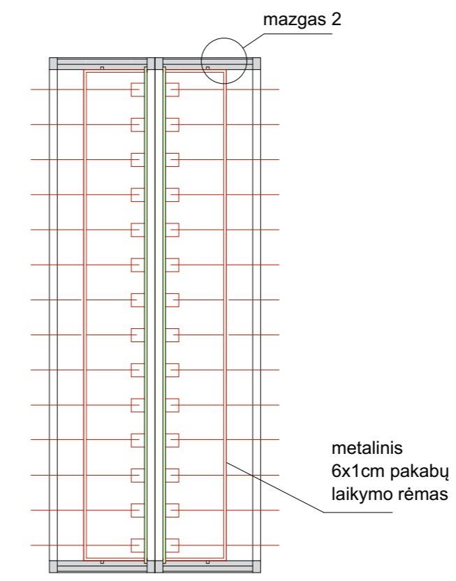
pjūvis 1-1
