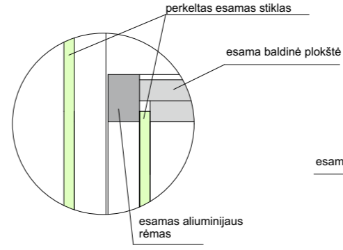
mazgas 4
