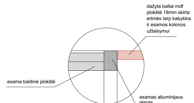
mazgas f
