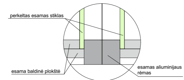
mazgas d
