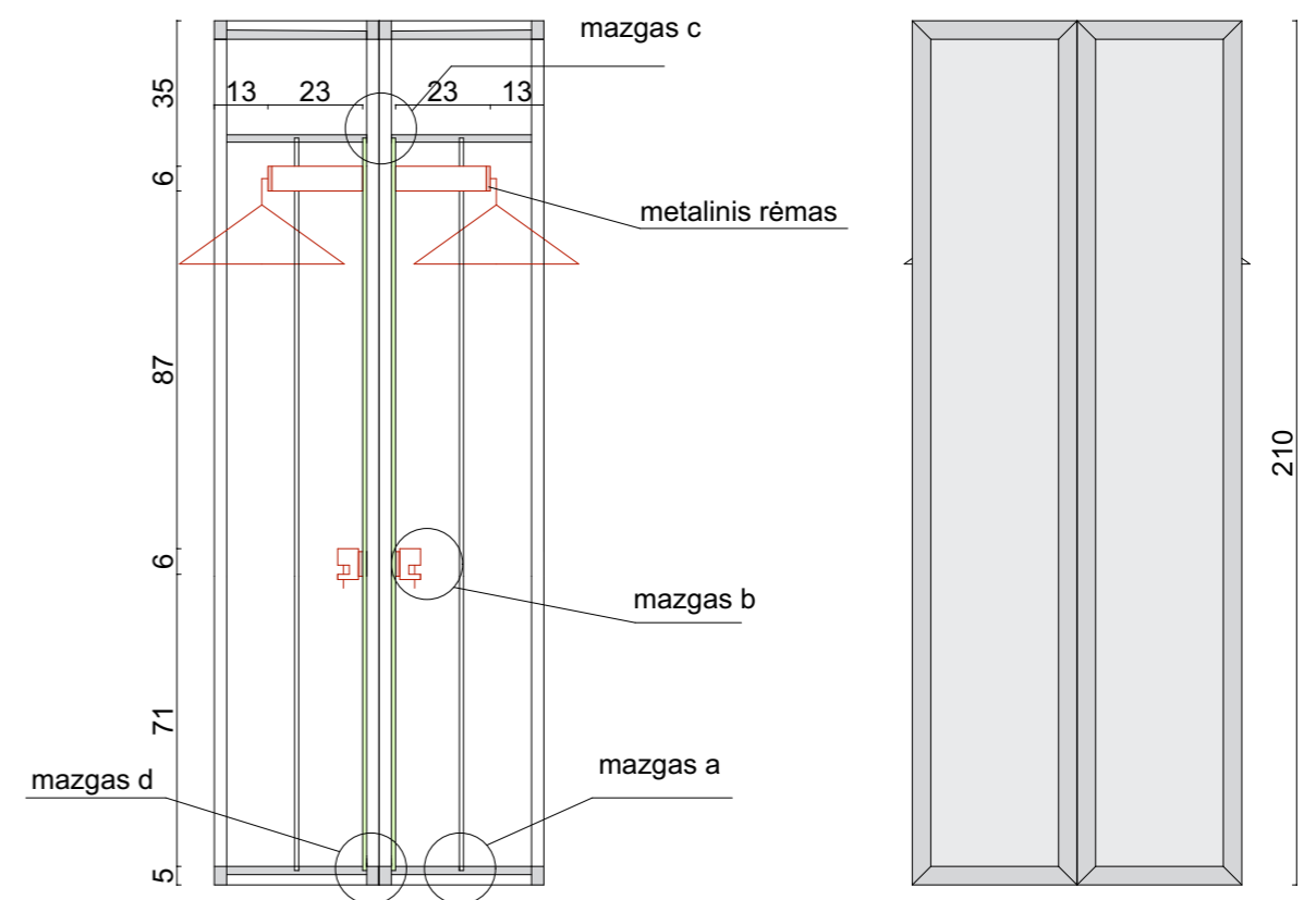
pjūvis 1-1
