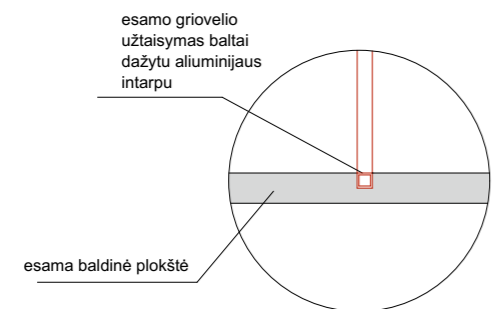
mazgas a
