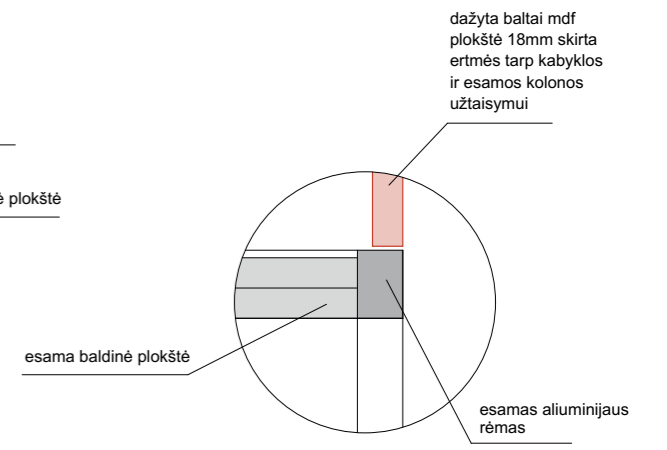
mazgas 5
