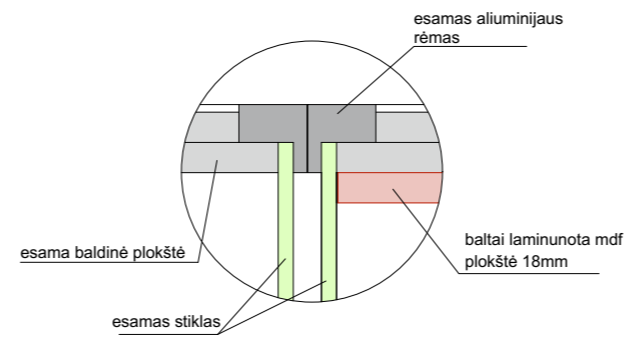
mazgas 2
