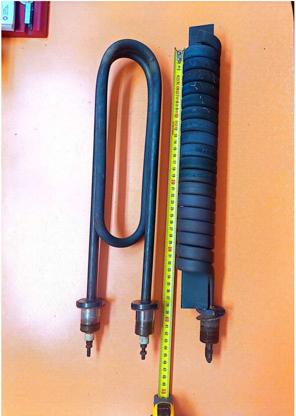
1 pav. Kaitinimo elementai: kairėje kaitinimo elementas Nr. 1, dešinėje kaitinimo elementas Nr. 2
