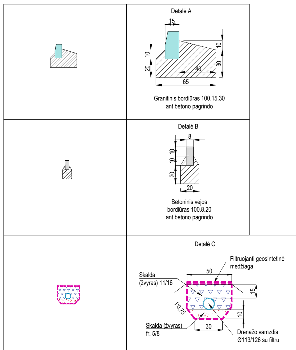
Detalių įrengimo schemos M 1:25 (Matmenys pateikti centimetrais)
