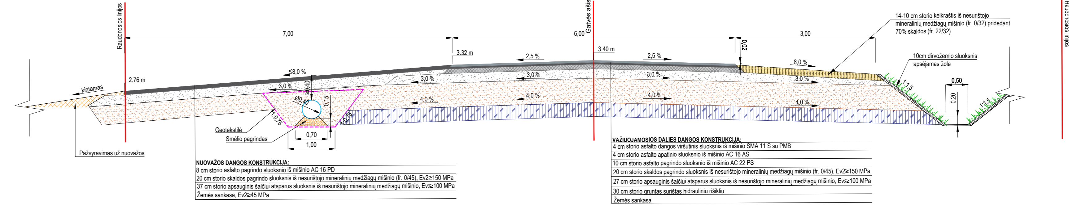
DANGOS KONSTRUKCIJOS SKERSINIS PROFILIS TIES NUOVAŽA PK 3+70
