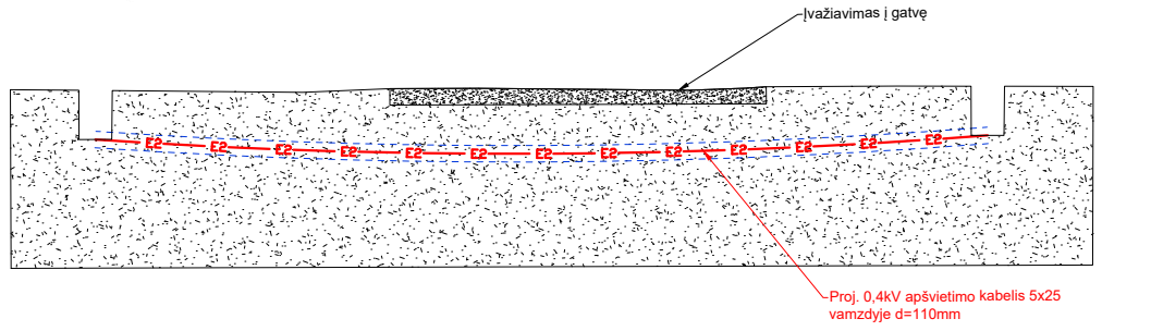
Ryšių kabelis ir projektuojamų elektros kabelių susikirtimų pjūvis
