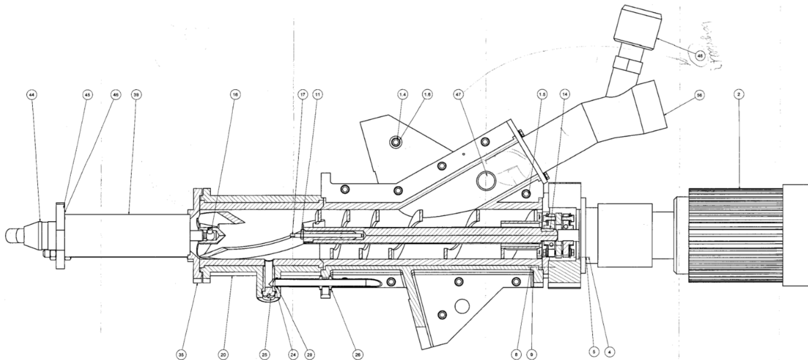
PRIEDAS Nr. 1 (D-4-D maišytuvo (mikserio) eskizas.)
