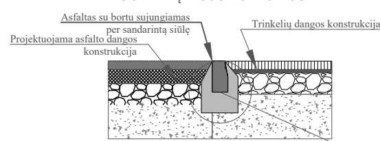
PROJEKTINIS IR ESAMO ŽVYRO/TRINKELIŲ DANGŲ KONSTRUKCIJŲ SLUOKSNIŲ SUJUNGIMO PJŪVIS
