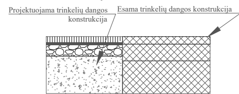
PROJEKTINIS TRINKELIŲ DANGŲ KONSTRUKCIJŲ SLUOKSNIŲ SUJUNGIMO PJŪVIS
