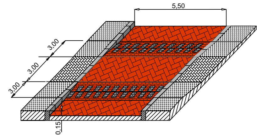
IŠKILIOS NEŽYMĖTOS PĖSČIŲJŲ PERĖJOS PRINCIPINĖ ĮRENGIMO SCHEMA
