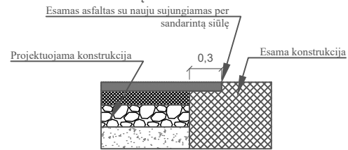
PROJEKTINĖS IR ESAMOS ASFALTO DANGŲ KONSTRUKCIJŲ SLUOKSNIŲ PERSIDENGIMO PJŪVIS
