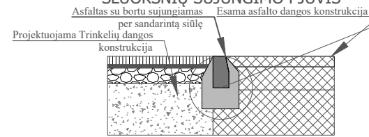
PROJEKTINIS TRINKELIŲ DANGŲ KONSTRUKCIJŲ SLUOKSNIŲ SUJUNGIMO PJŪVIS
