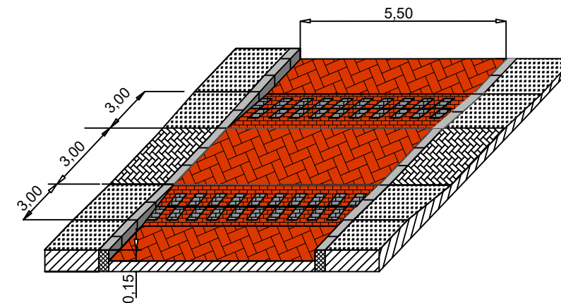
IŠKILIOS NEŽYMĖTOS PĖSČIŲJŲ PERĖJOS PRINCIPINĖ ĮRENGIMO SCHEMA
