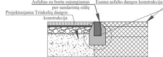
PROJEKTINIS TRINKELIŲ DANGŲ KONSTRUKCIJŲ SLUOKSNIŲ SUJUNGIMO PJŪVIS
