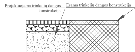
PROJEKTINIS TRINKELIŲ DANGŲ KONSTRUKCIJŲ SLUOKSNIŲ SUJUNGIMO PJŪVIS
