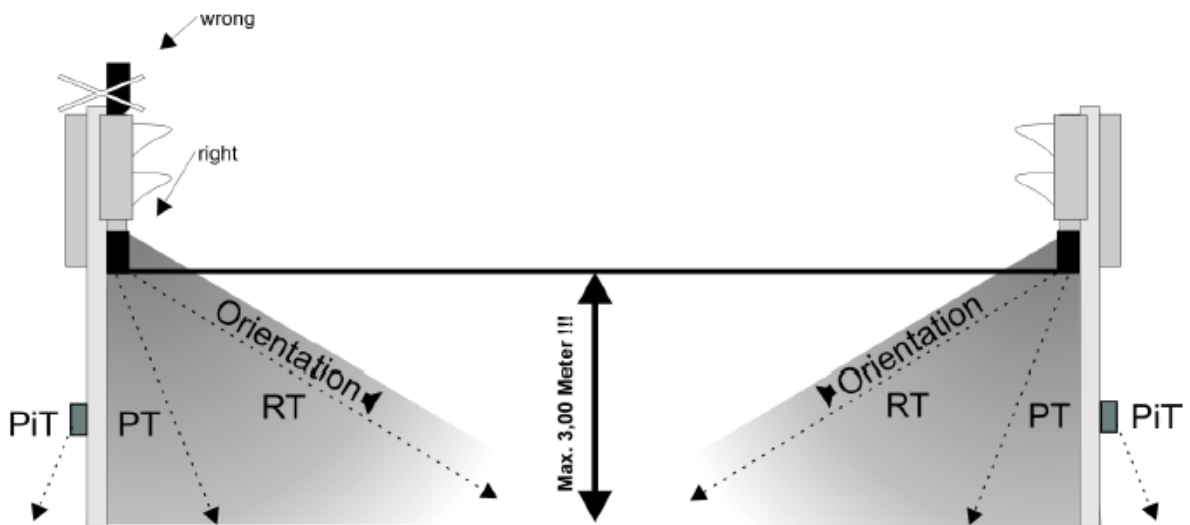
1 pav. Akustinių įrenginių ir mygtukų įrengimo pavyzdys
