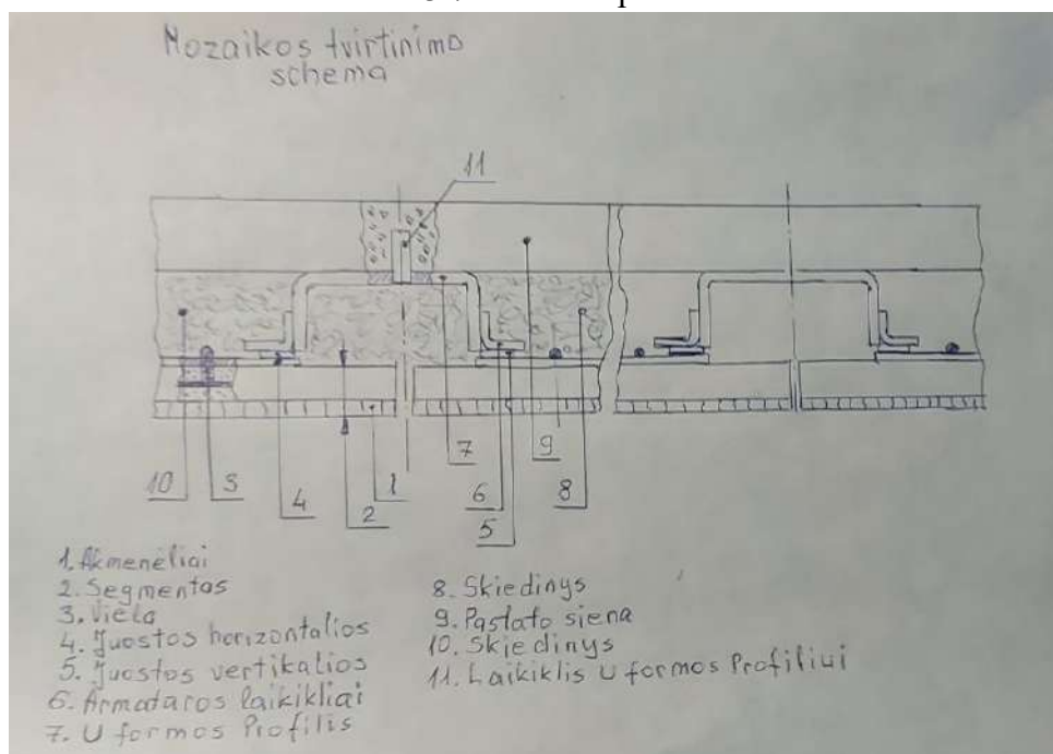
Pav. 3.8 Principinė tvirtinimo schema
