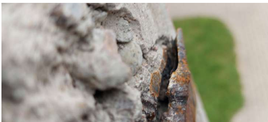
Pav. 8.5 Atitrūkų suvirinimo taškai
