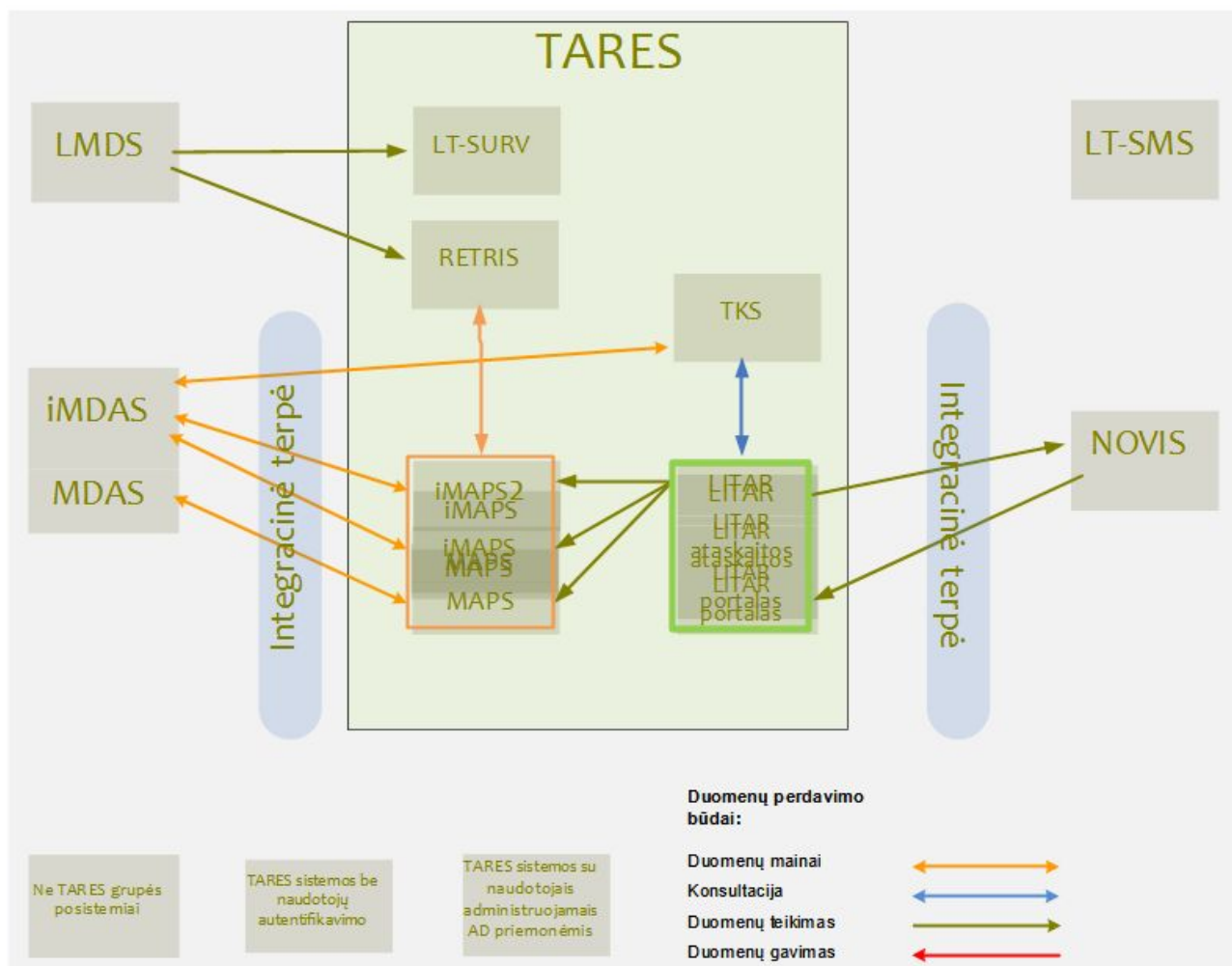
7 pav. TARES sistemų tarpusavio sąsajos ir sąsajos su kitomis integruotos MIS
