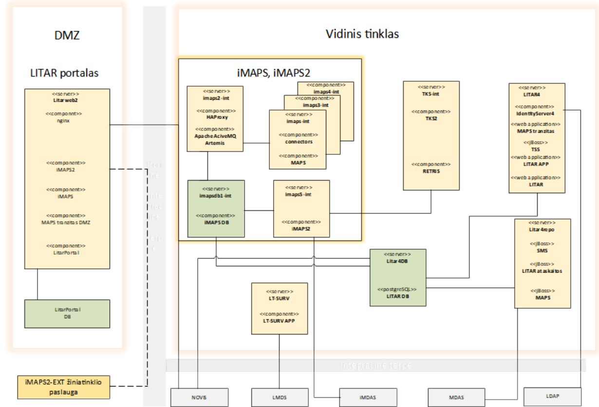
9 pav. Bendroji TARES techninė architektūra
