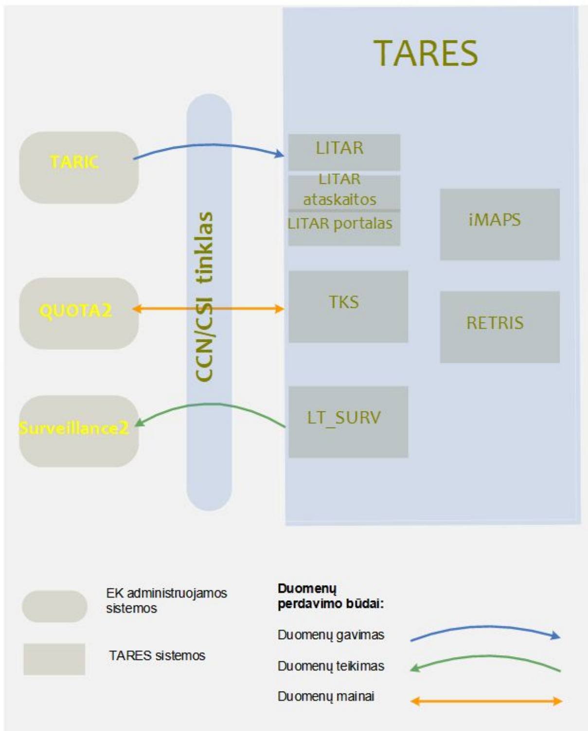
8 pav. TARES sąsajos su išorinėmis informacinėmis sistemomis
