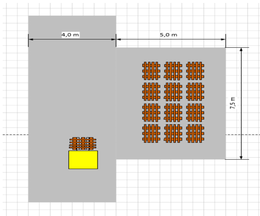
2 pav. Preliminari statinio schema
