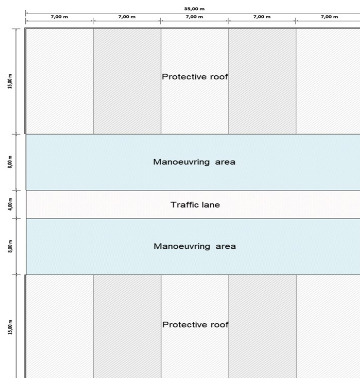
1 pav. Preliminari statinio schema
