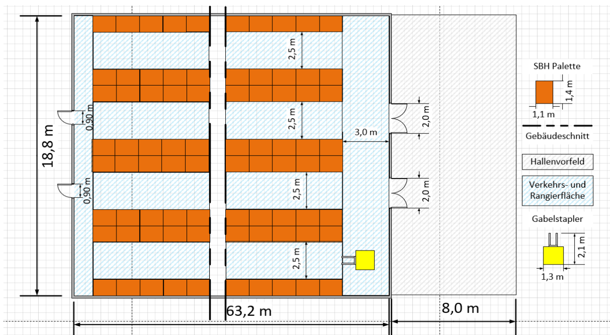
1 pav. Preliminari sandėliavimo patalpos schema
