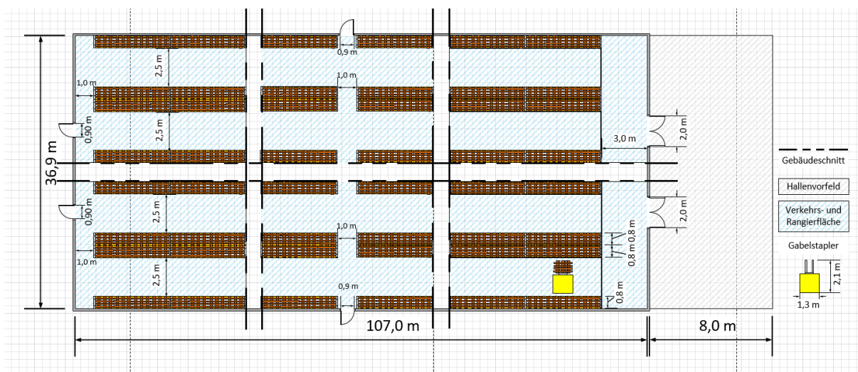
1 pav. Preliminari sandėliavimo patalpos schema
