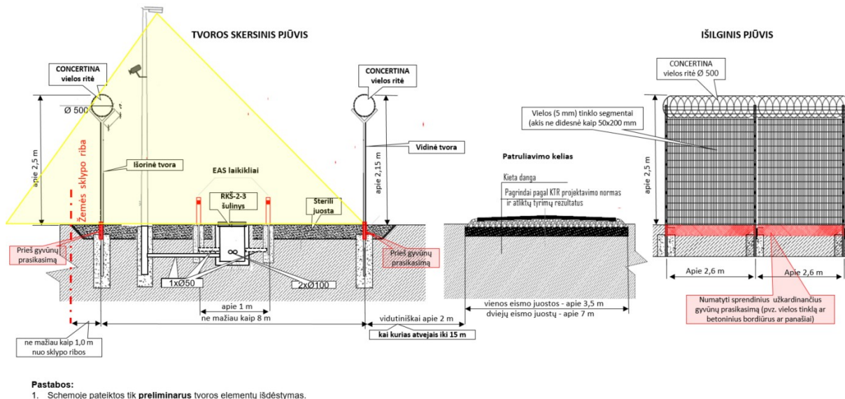
1 pav. Tvoros elementų preliminarus išdėstymo skersiniame pjūvyje schema
