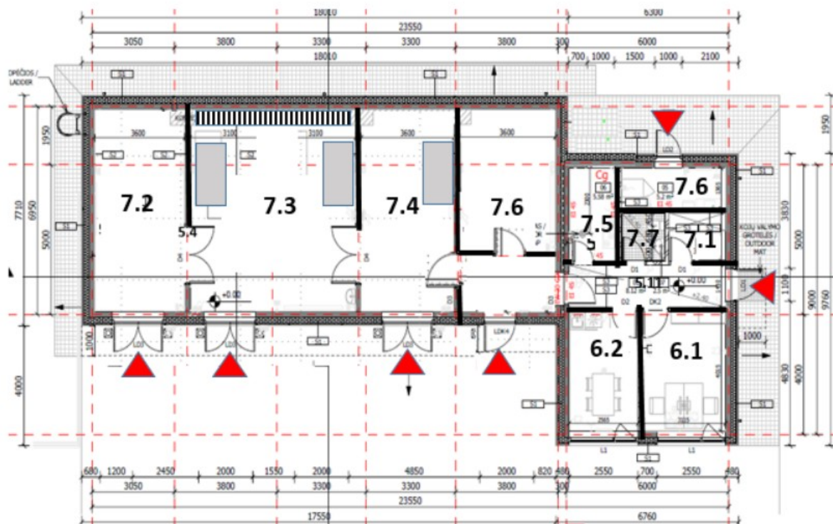
1 pav. Preliminari statinio schema
