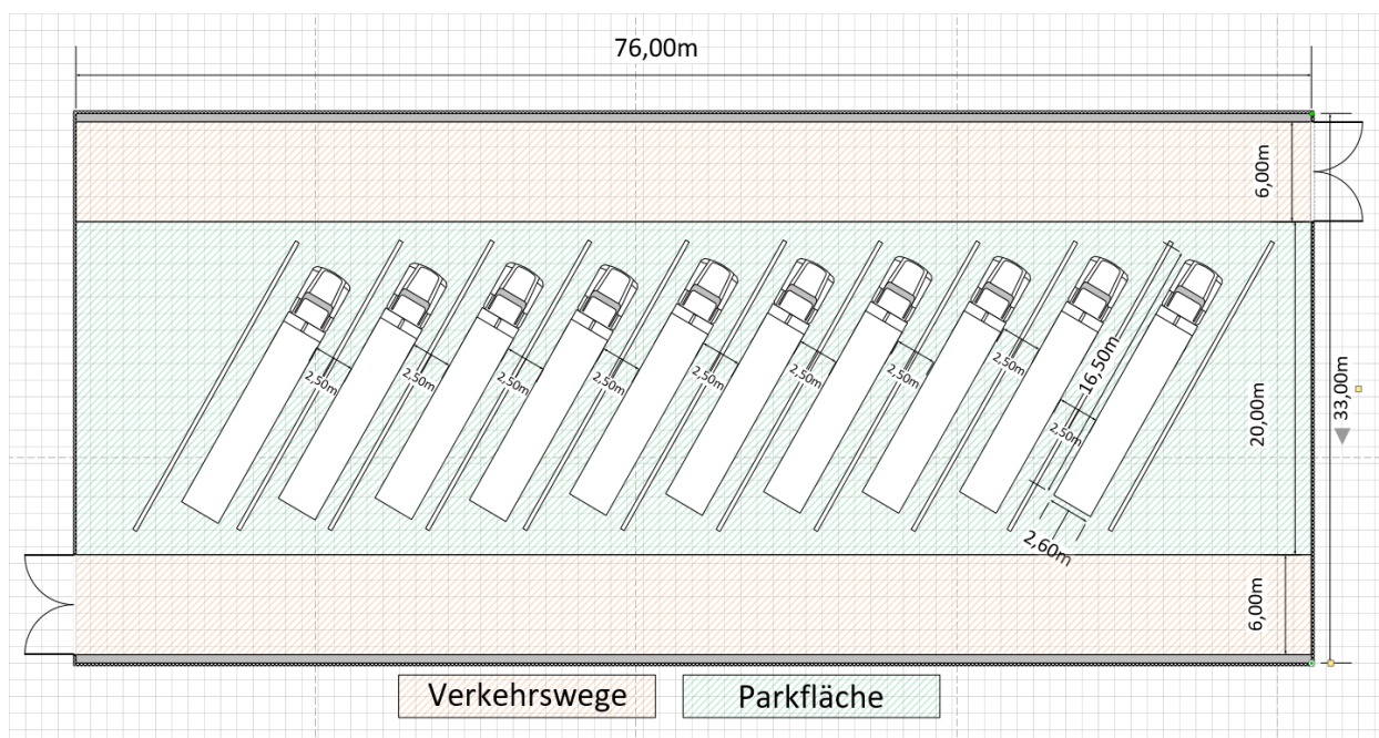
1 pav. Aikštelės preliminarus išdėstymo schema.
