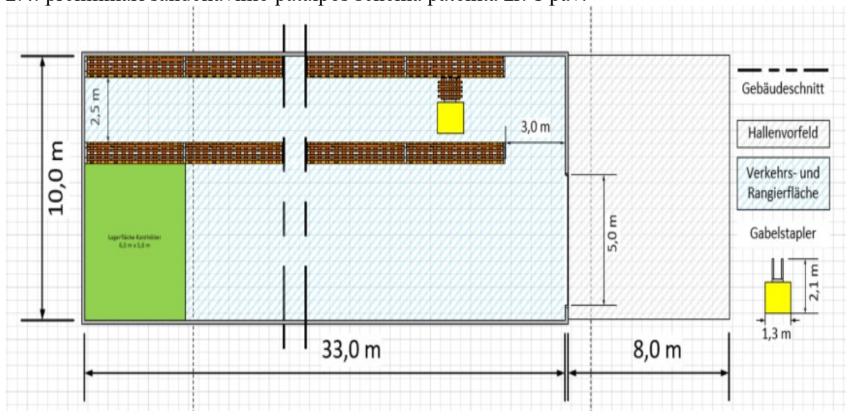
1 pav. Preliminari sandėliavimo patalpos schema
