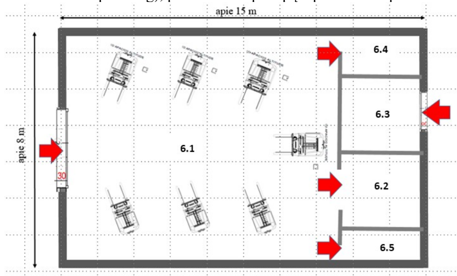
1 pav. Preliminarus elektrinių krautuvų garažo išplanavimas ir funkciniai ryšiai
