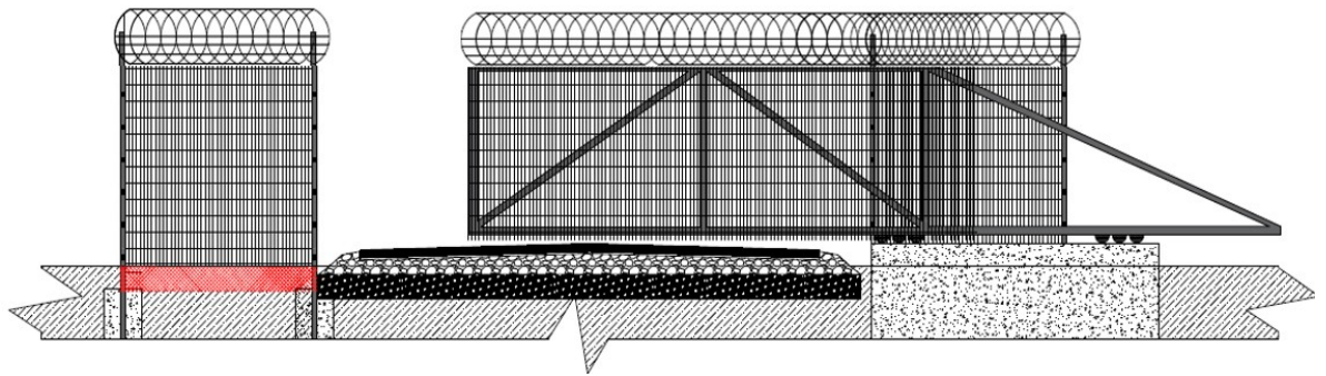
2 pav. Tvoros vartų preliminarinė schema
