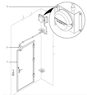
2 pav. Informacinio šviestuvo įrengimo vizualizacija
