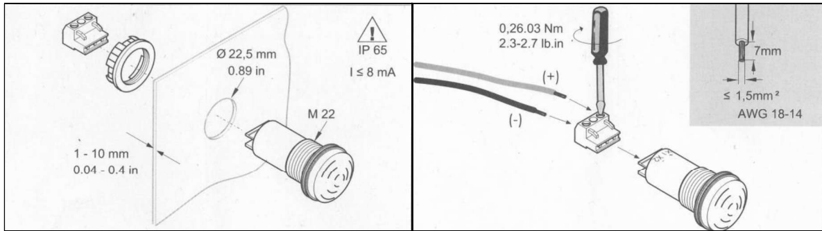
Garsinio signalo akliems montavimo šviesoforo korpuse schema
