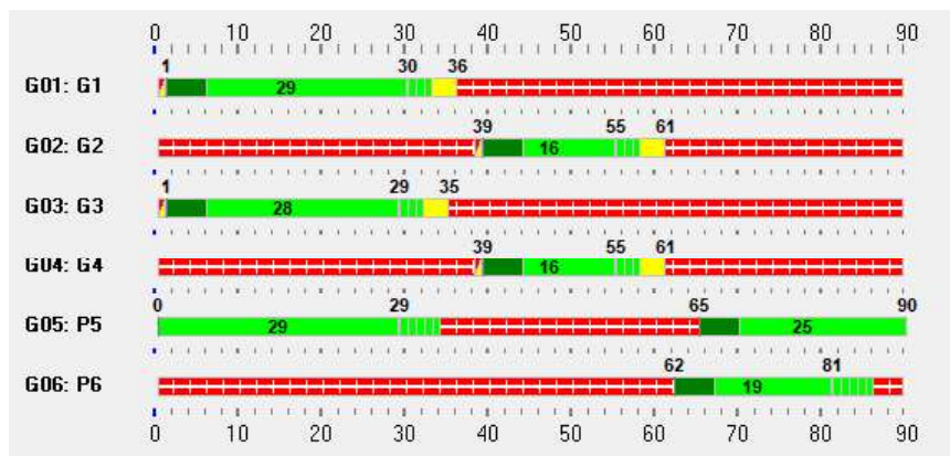
Šviesoforų valdiklio fiksuotas darbo režimas
