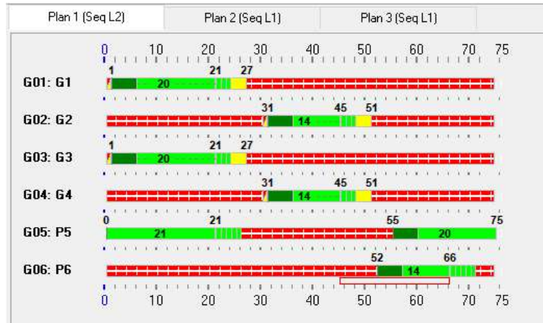
Šviesoforų valdiklio darbo režimas
