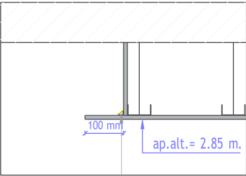
Mazgas a-a M1:10
