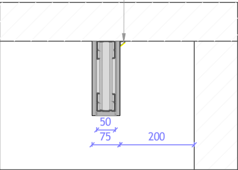
Mazgas b-b M1:10
