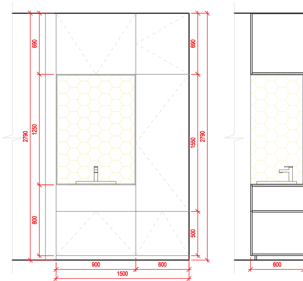
sp-9- Spinta su praustu- drabužinė su praustuvo spintele nišoje; LMDP
