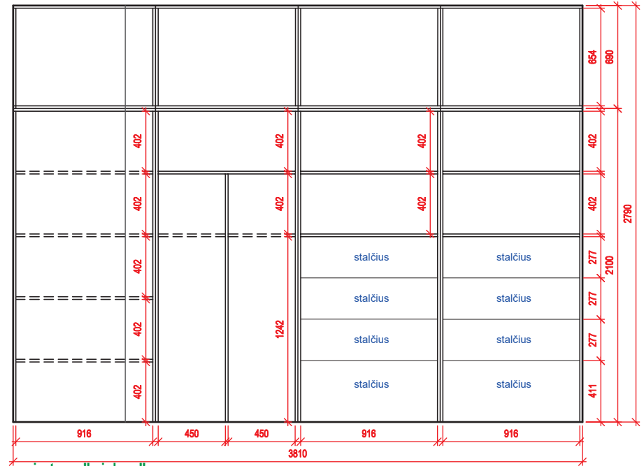
spintos "vidus"
