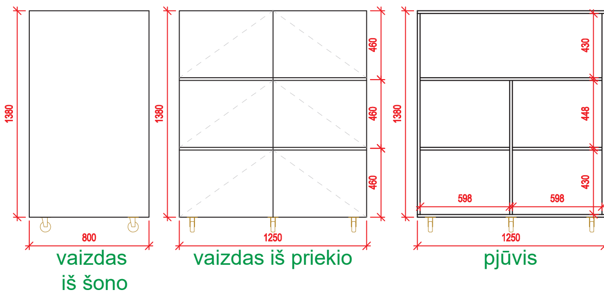
sp-3- inventoriaus spintelė- spintelė-tumba ant ratukų su 3-jomis atverčiamomis durelėmis; LMDP
