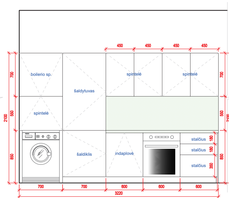
išklotinė V2
