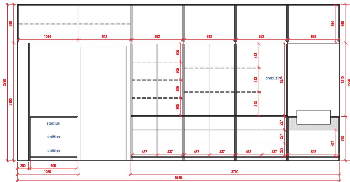
spintos "vidus"
