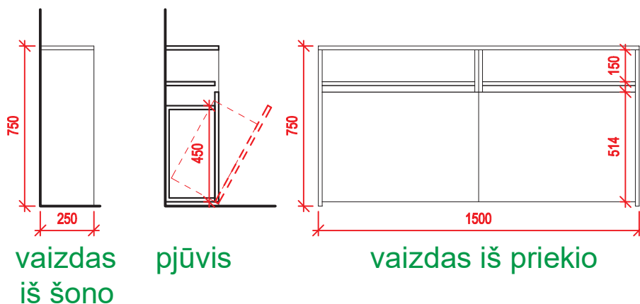
sp-6- spintelė "LENTA"- dvi atverčiamos durelės-pakylės; LMDP
