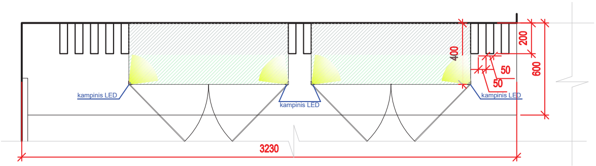
pjūvis
