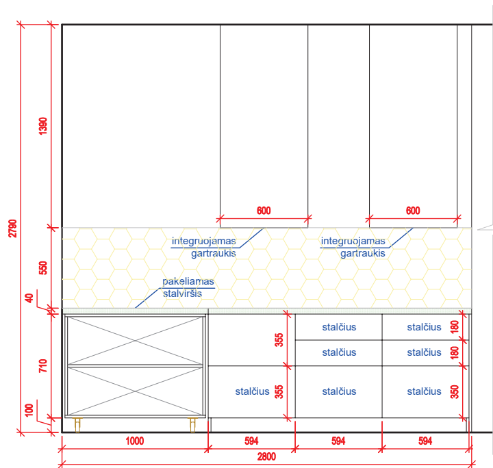
išklotinė V1
