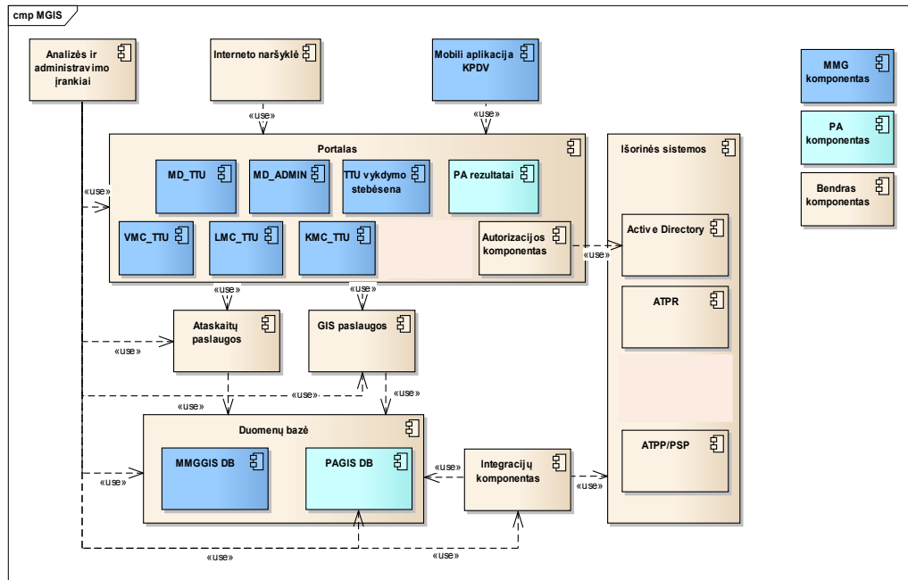
6 pav. MGIS funkcinė architektūra ir integracinės sąsajos
