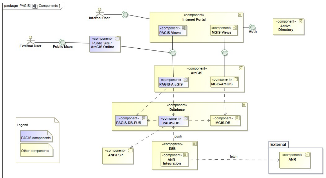
7 pav. Loginiai sistemos komponentai
