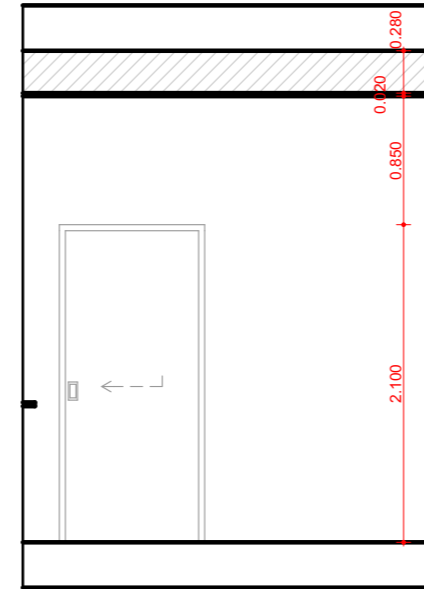
003 02 1:50
