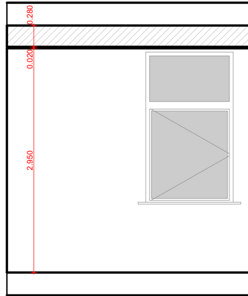
003 01 1:50
