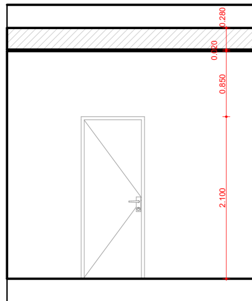
003 03 1:50
