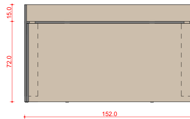
Pjūvis - 1
