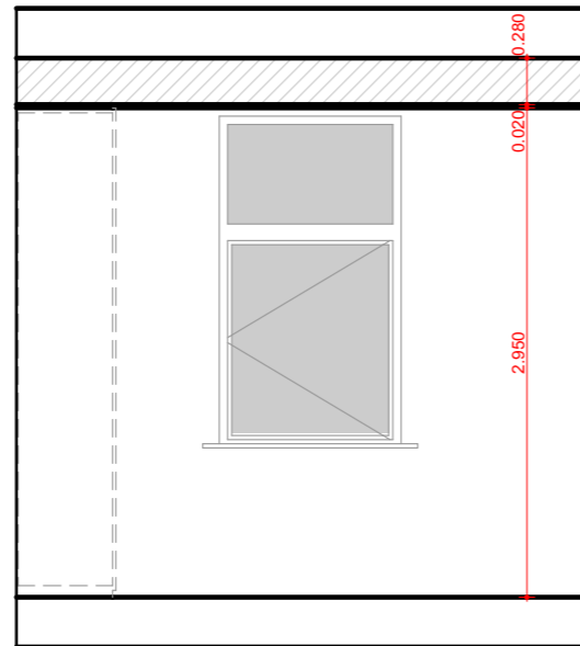
007 03 1:50
