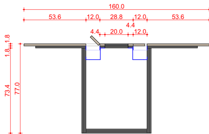
Pjūvis 1-1
