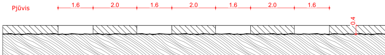
Rašto schema M 1:5
