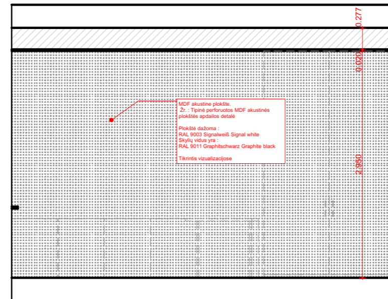
005 02 1:50
