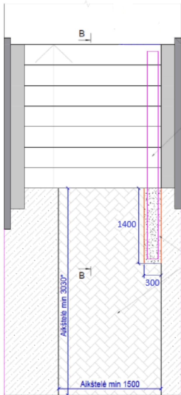
Vaizdas iš viršaus A-A
