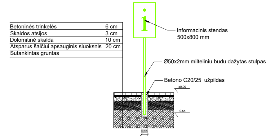
STENDO ĮRENGIMO DETALĖ
