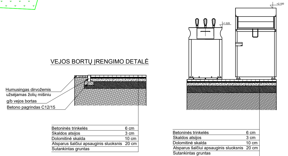
AIKŠTELĖS DANGOS KONSTRUKCIJA
