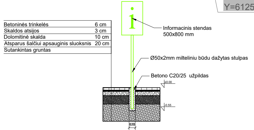
STENDO ĮRENGIMO DETALĖ
