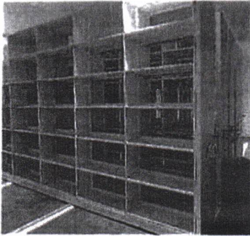
Mobilus dvipusis stelažas - 4500x600x2800 (h) mm Spalva – šviesiai pilka RAL 7035,
