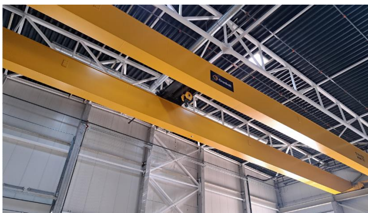
12. Pav. Dvisijos tiltinis kranas CRANBALT, gamyklinis Nr. 24-074
