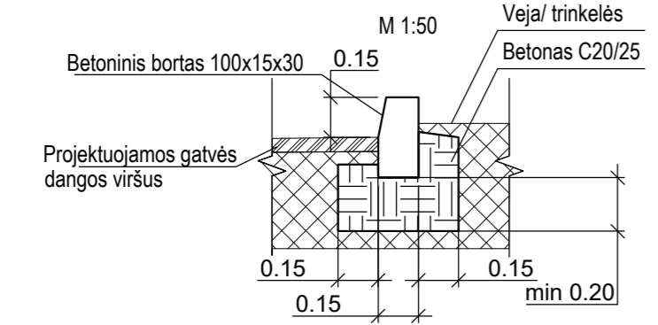
Gatvės bordiūras 100x15x30 M 1:50
