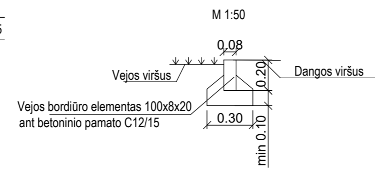
Vejos bordiūras 100x8x20 M 1:50
