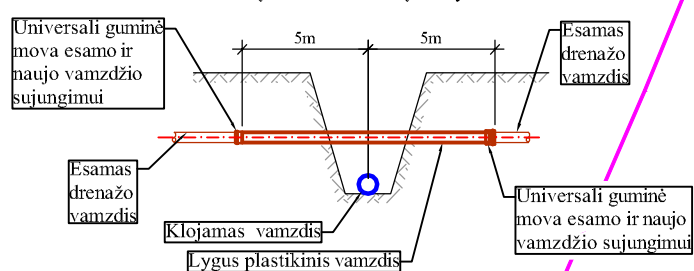
Pažeistų drenažo rinktųjų atstatymo detalė
