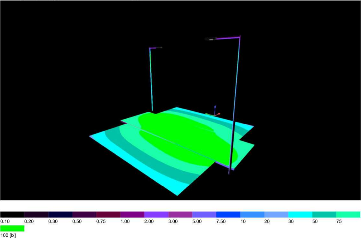
Trakai, perėjos (2), Illuminance values in [lx]
