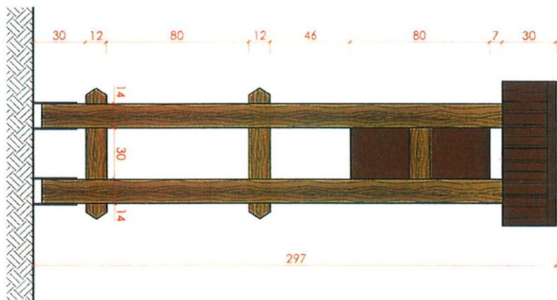
VAZDAS IŠ GALO, M 1:20
