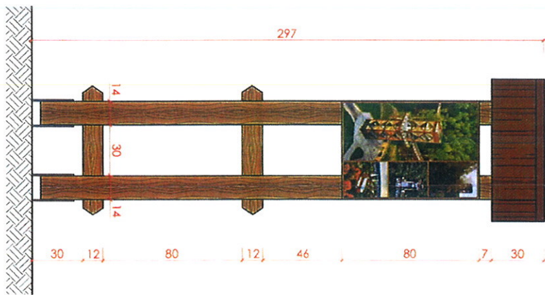
VAZDAS IŠ PRIEKIO, M 1:20
