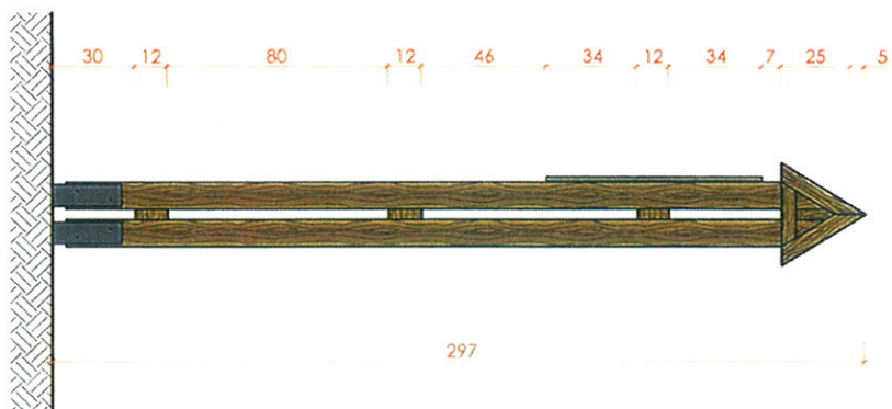
VAZDAS IŠ ŠONO, M 1:20
