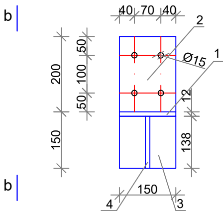
Detalė D-2 M 1:10
