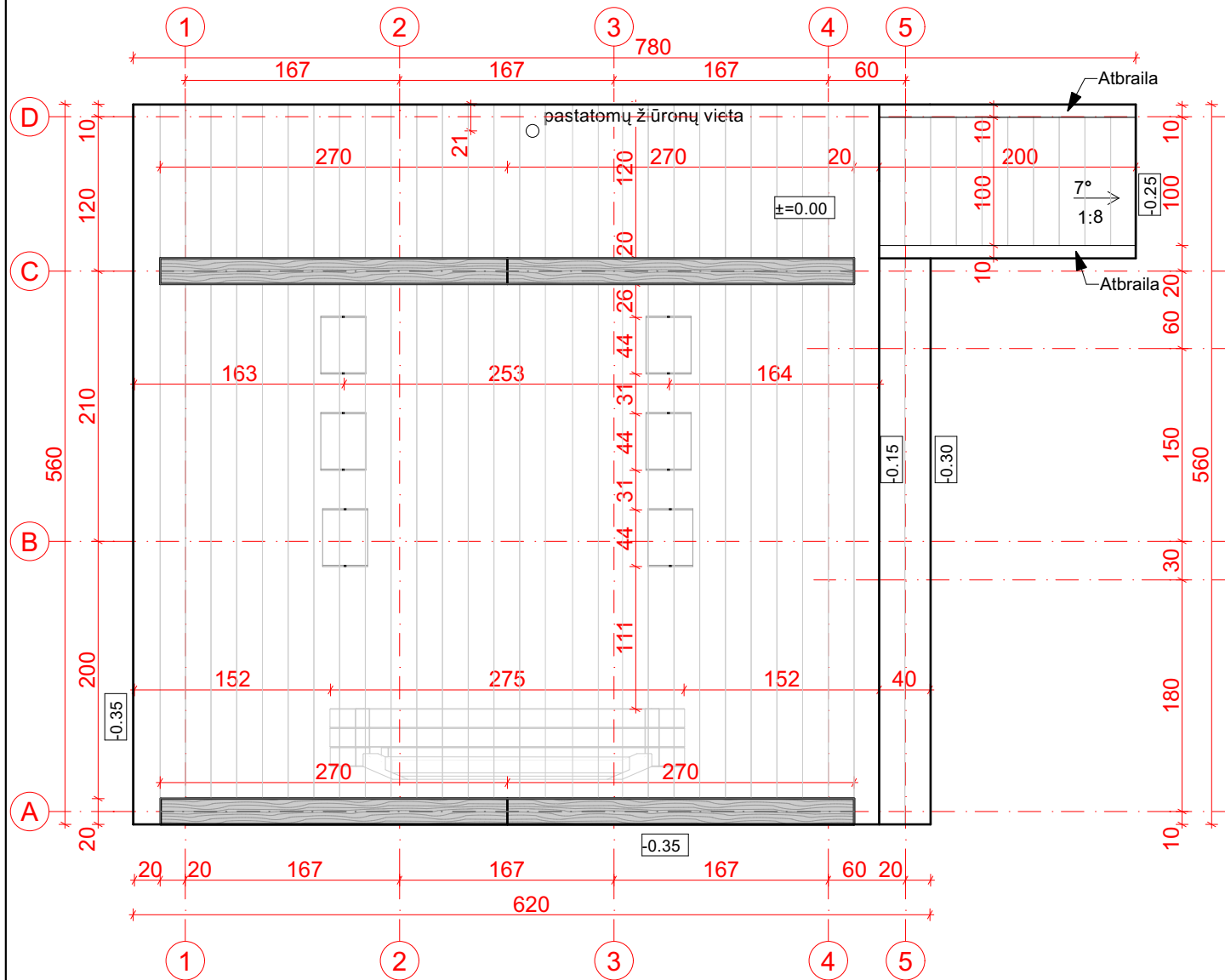
Apžvalgos aikštelės planas 1:50
