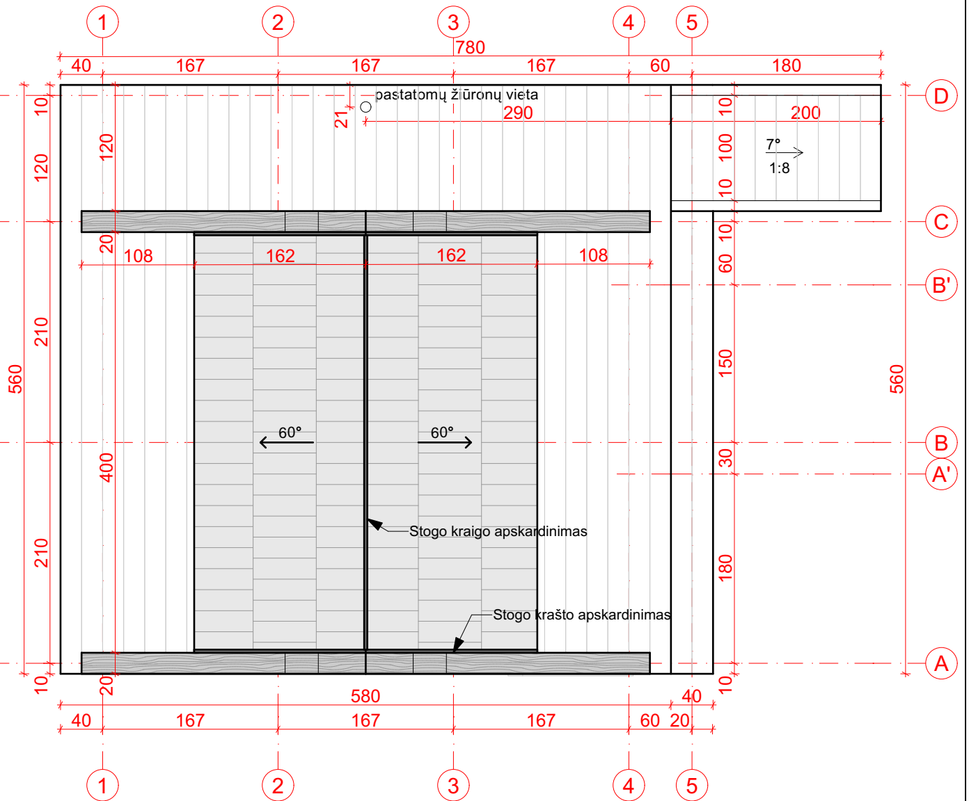
Apžvalgos aikštelės stogo planas 1:50
