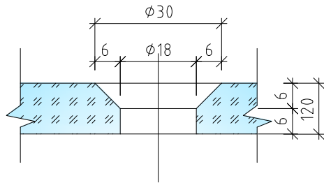
PJŪVIS PER SKYLĘ STIKLE
