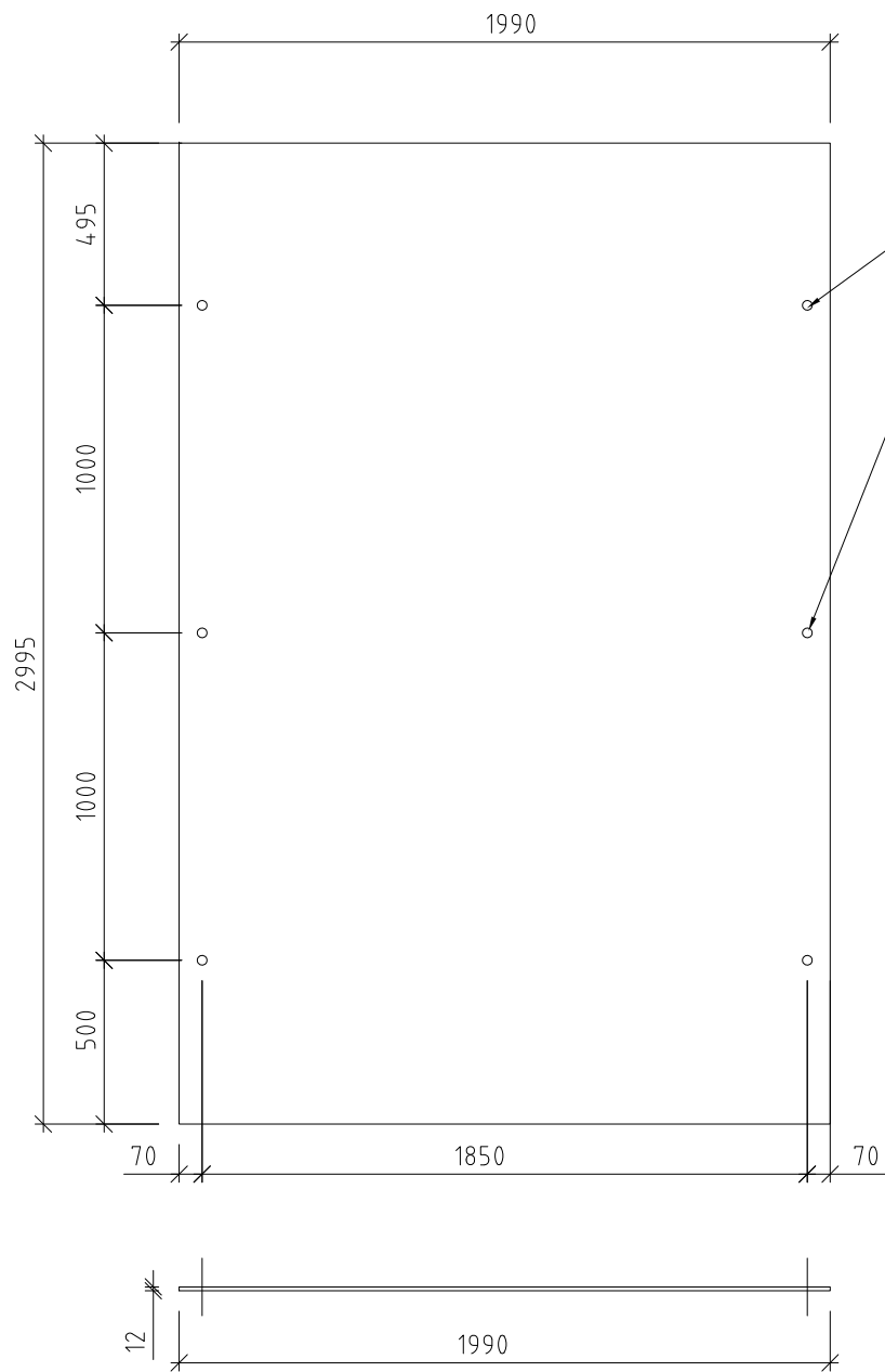
STIKLO LAKŠTAS Nr.1
