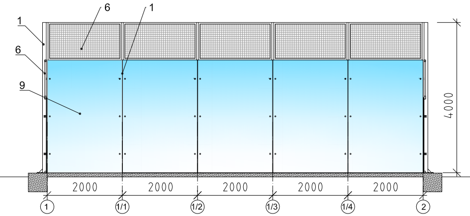
PJŪVIS A-A M 1:100
