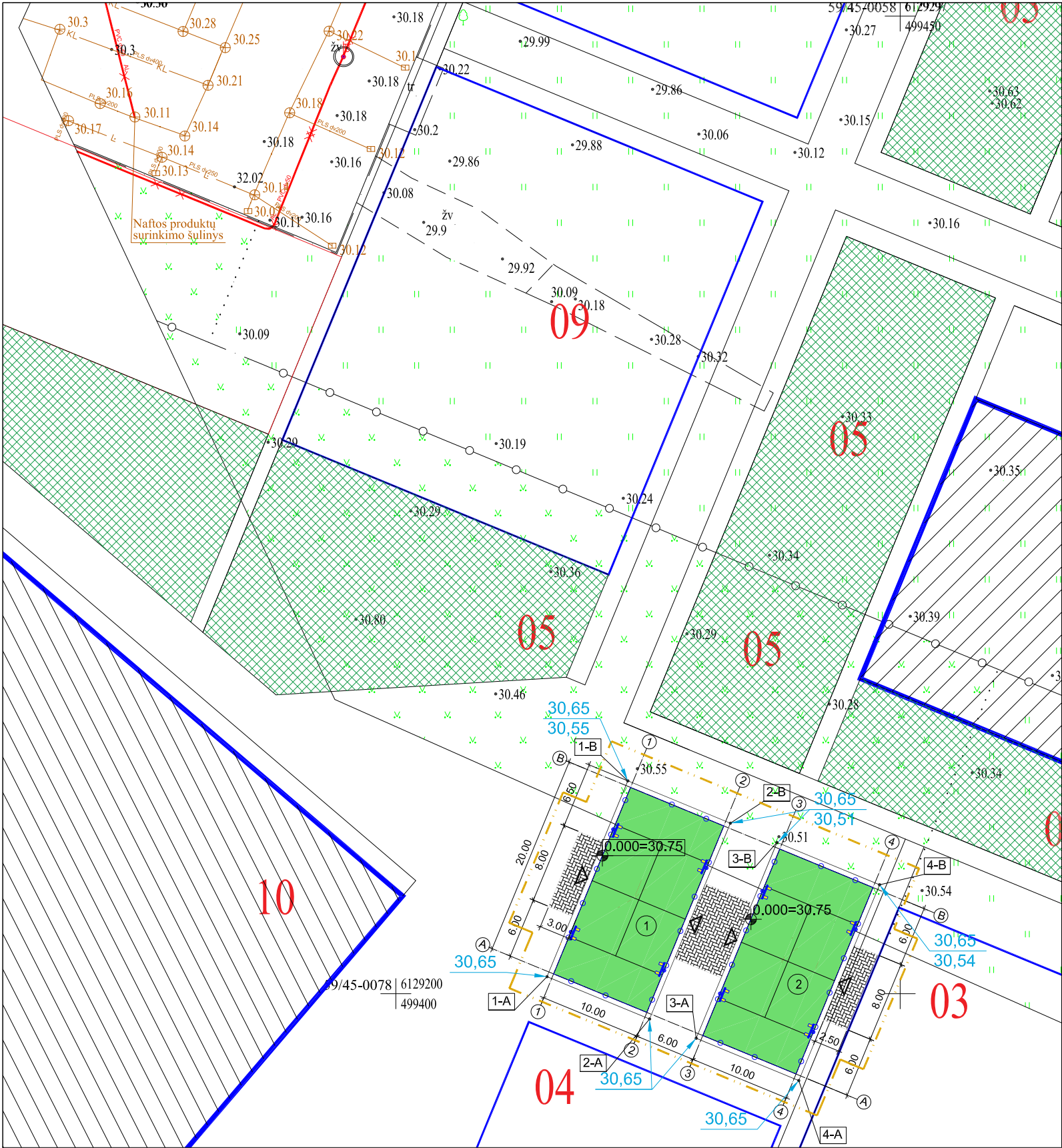
SKLYPO OBJEKTŲ EKSPLIKACIJA
