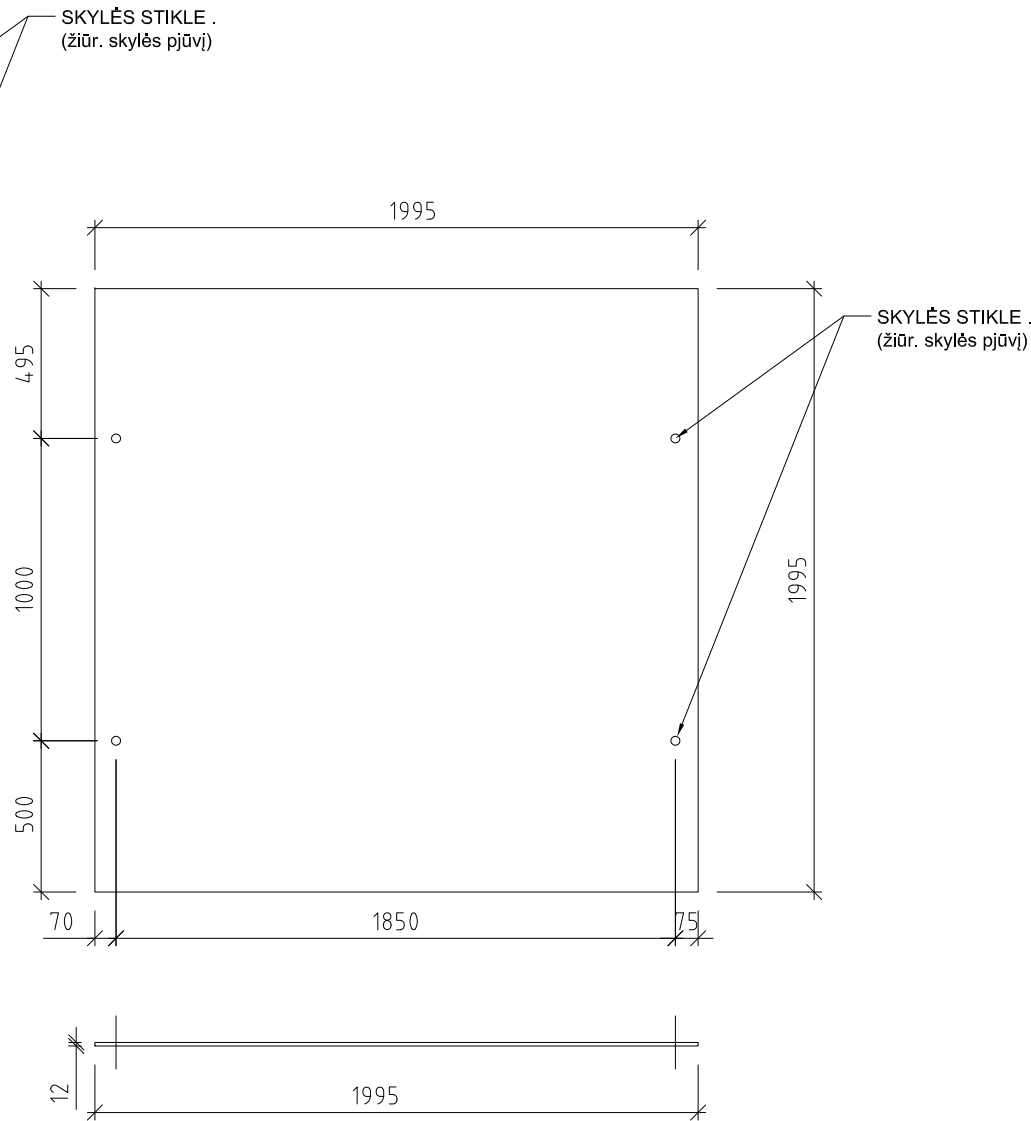
STIKLO LAKŠTAS Nr.2
