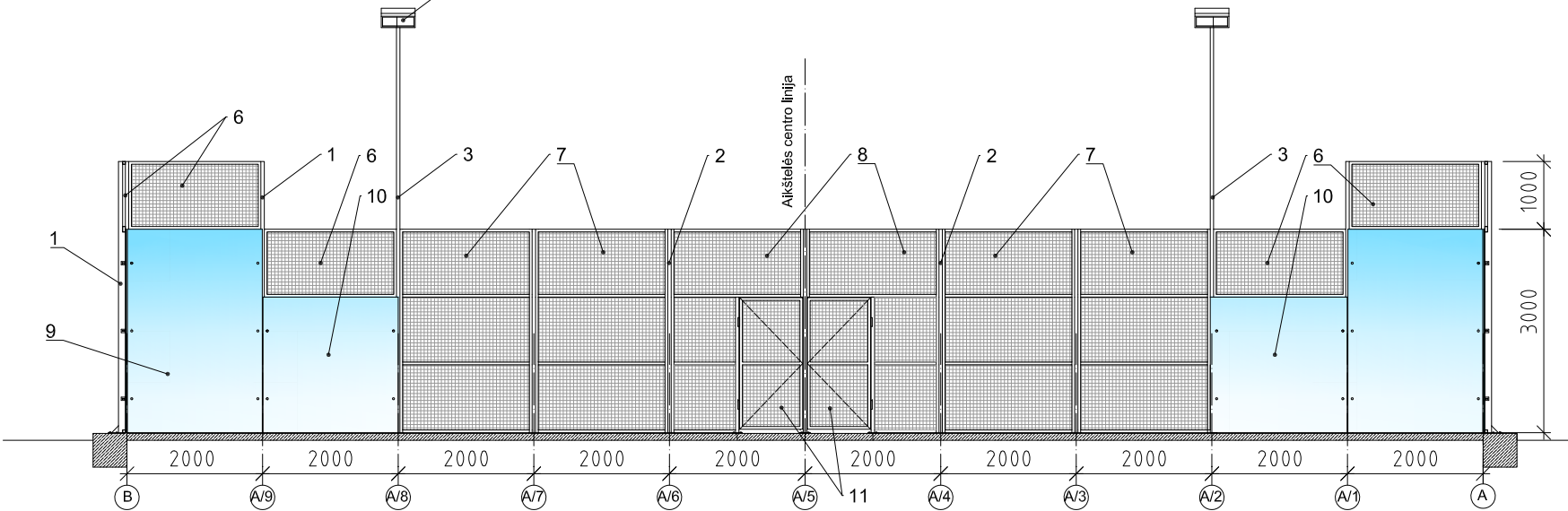
IŠKLOTINĖ TARP AŠIŲ B-A M 1 2 :100
