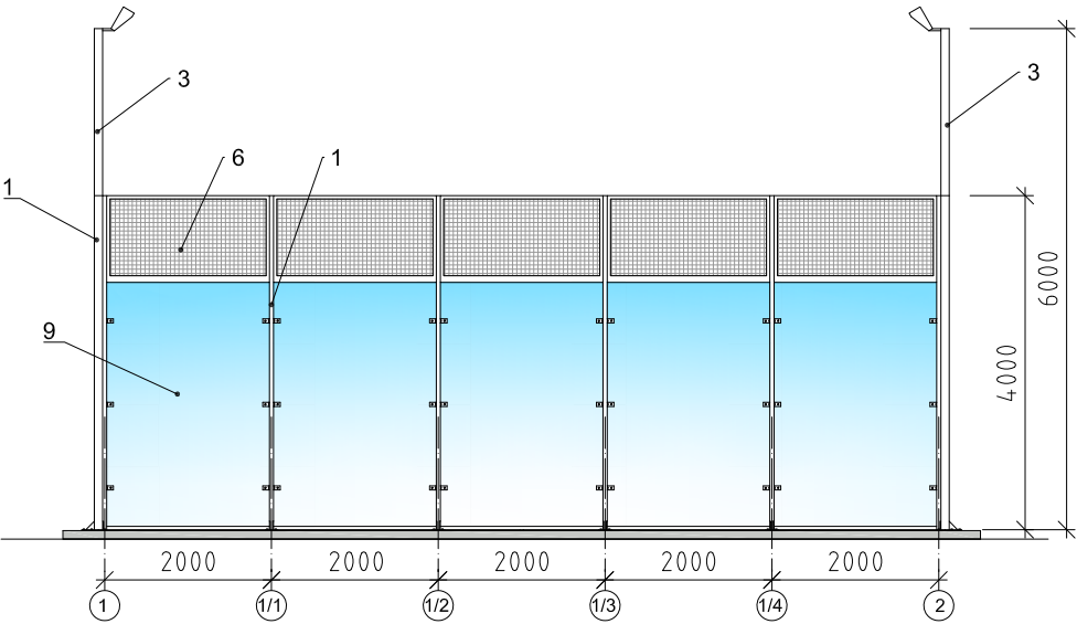
IŠKLOTINĖ TARP AŠIŲ 1-2 M 1:100
