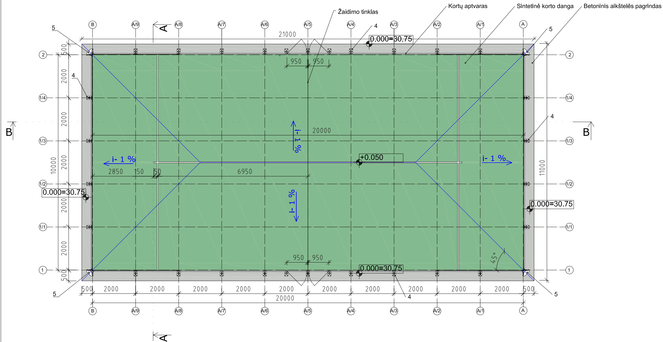
AIKŠTELĖS SU APTVARU PLANAS
