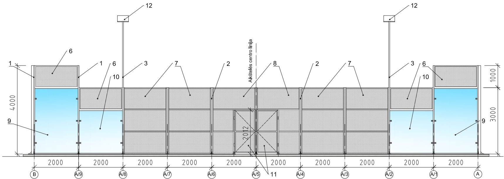
IŠKLOTINĖ TARP AŠIŲ B-A M 1 2 :100
