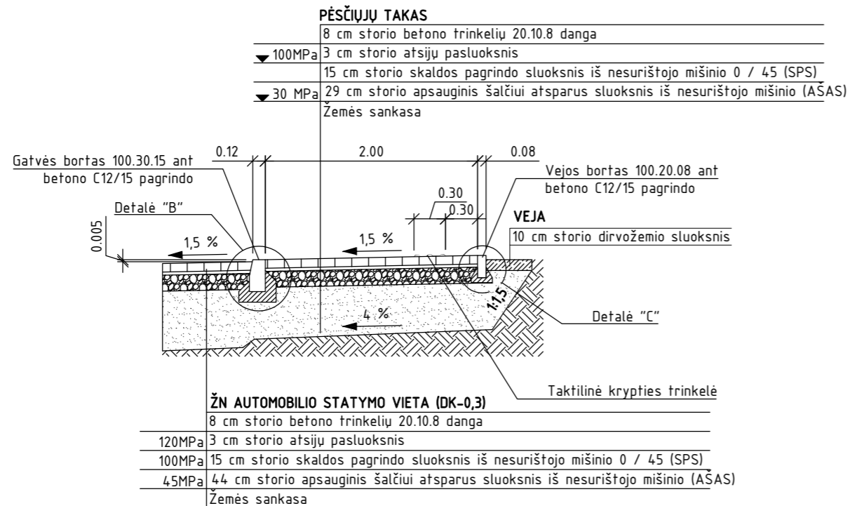
Skersinis pjūvis "2-2"; M1:50
