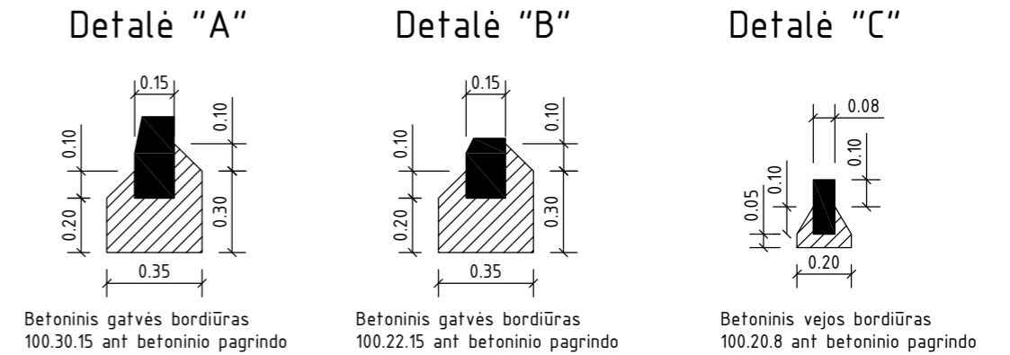
Bortū jrengimo schema M1:25
