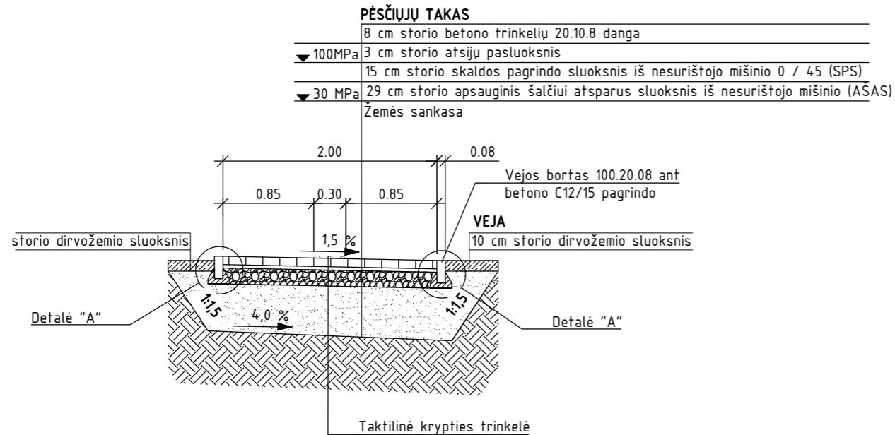
Skersinis pjūvis "1-1"; M1:50
