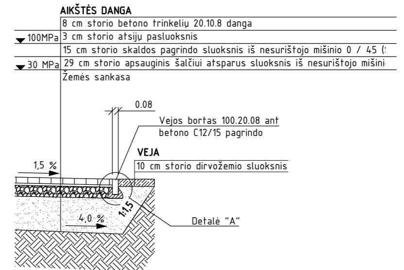
Skersinis pjūvis "3-3"; M1:50
