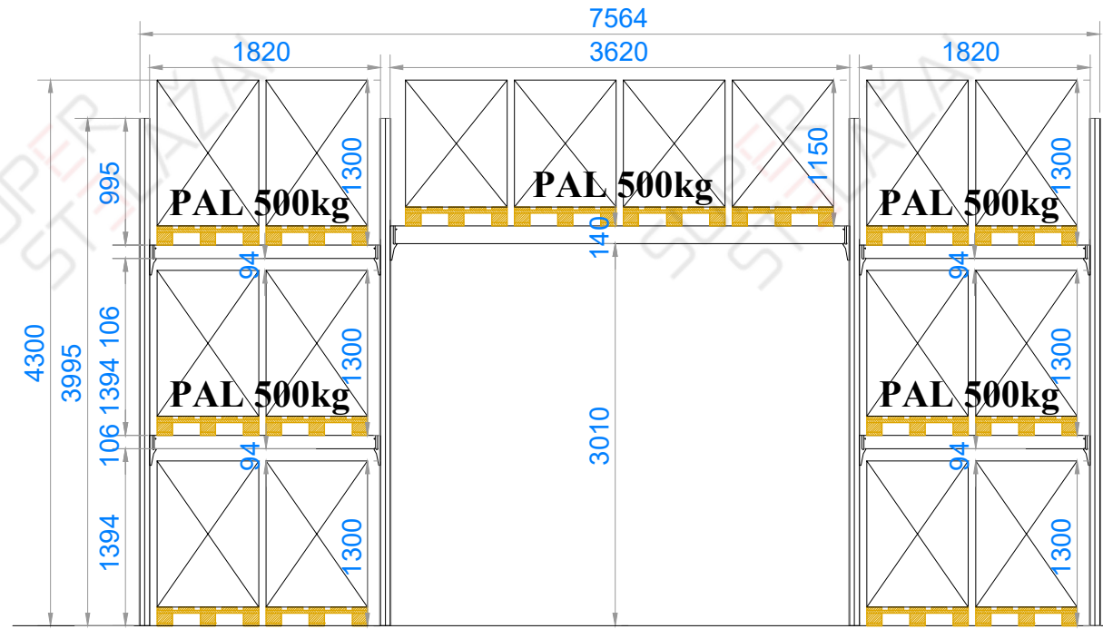
Pjūvis A-A
