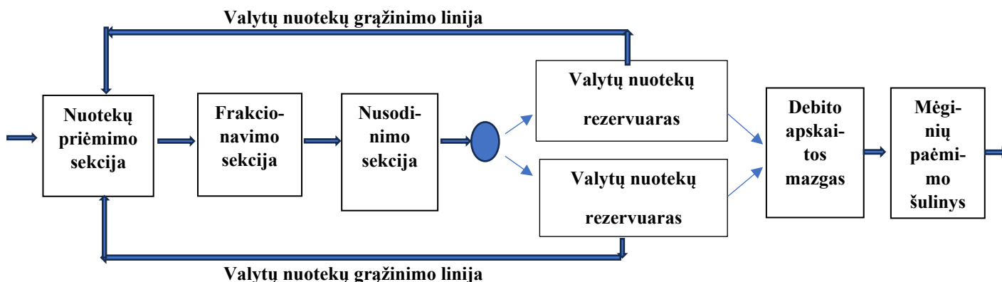
3 pav. Nuotekų valymo proceso schema
